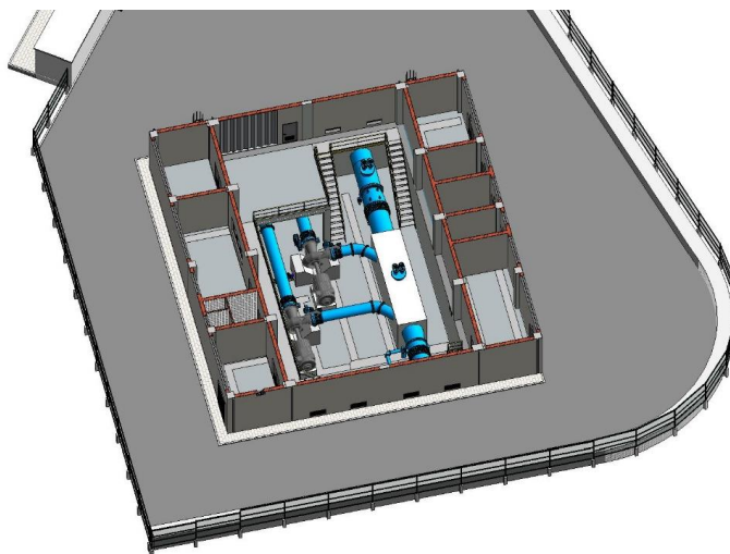
Figura 4.5 – Modelo BIM da CH de Ervidel-Sado. Vista do interior da Central.
