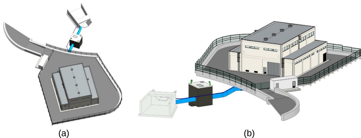
Figura 4.4 – Modelo BIM da CH de Ervidel-Sado. Vistas exteriores.
