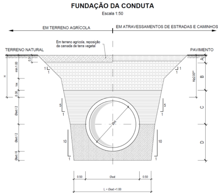
Figura 4.1 – Vala tipo para instalação da conduta adutora
