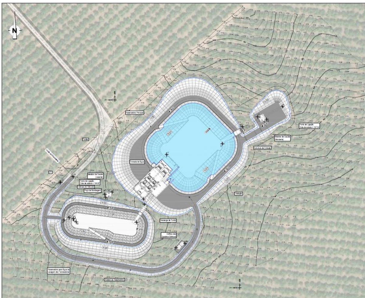
Figura 4.3 – Camara de Carga (planta).
