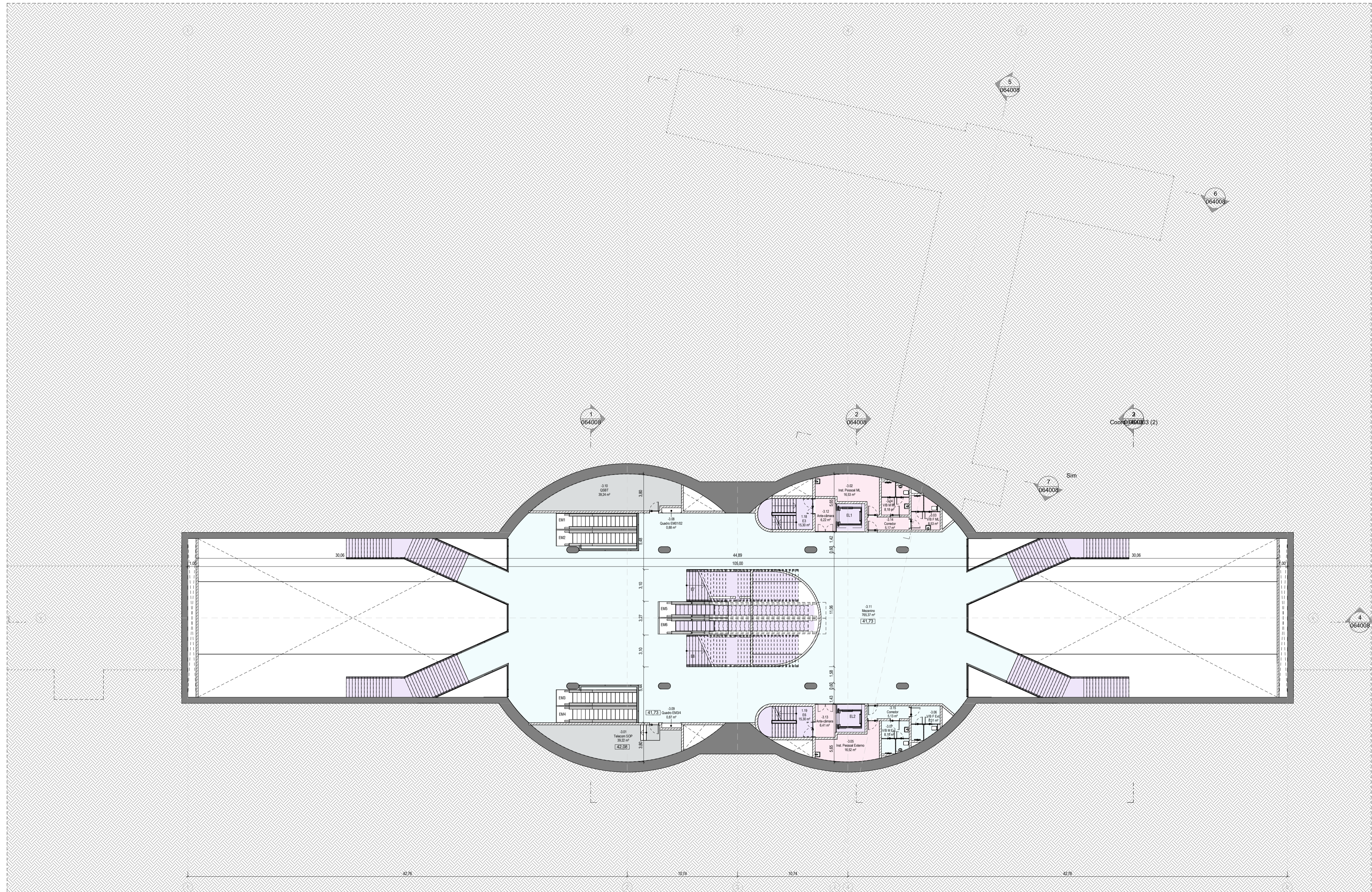
PLANTA DO MEZANINO 1 : 200
