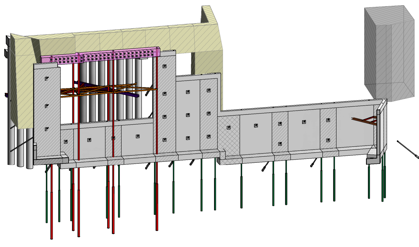
VISTA 3D - ALÇADO CD s / escala
