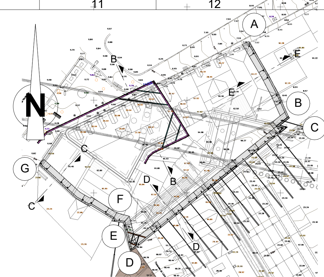
PLANTA DE DIMENSIONAMENTO IDENTIFICAÇÃO DOS CORTES Esc. 1 : 500
