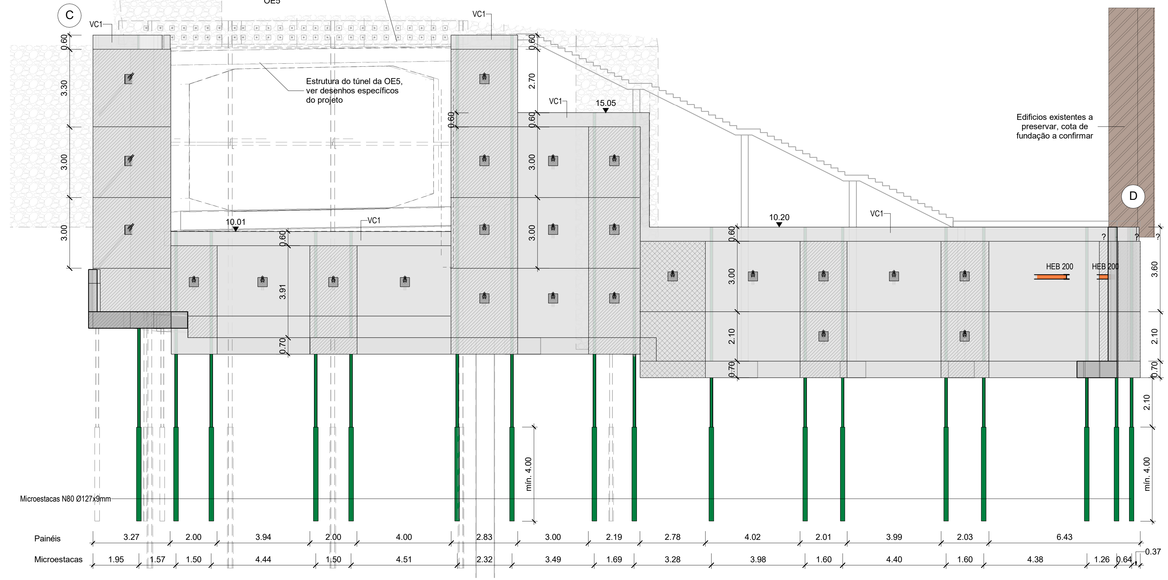
ALÇADO CD Esc. 1 : 100
