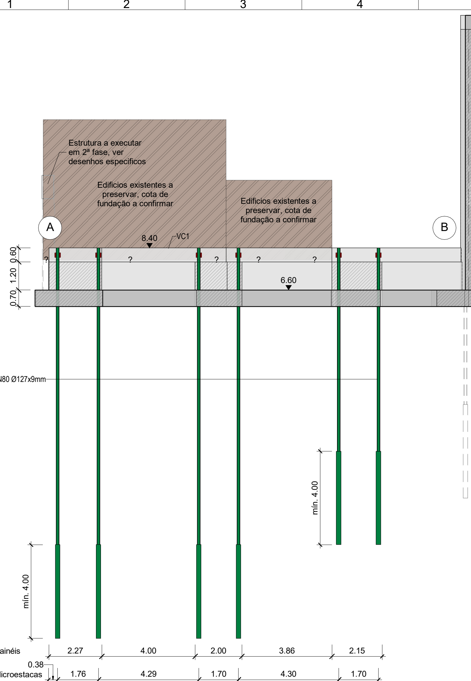
ALÇADO AB Esc. 1 : 100
