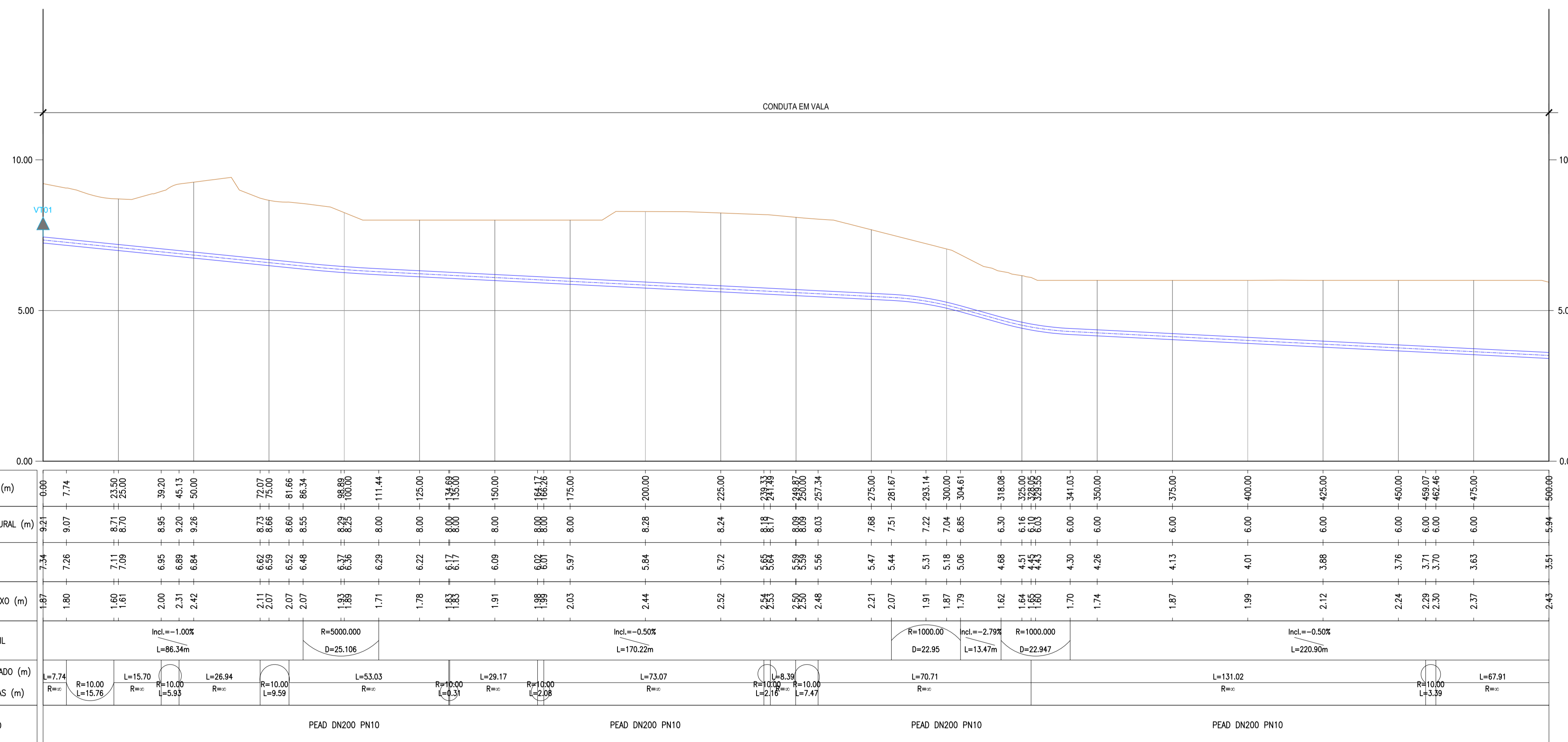
PERFIL LONGITUDINAL ESCALA: H=1:1000;V=1:100
