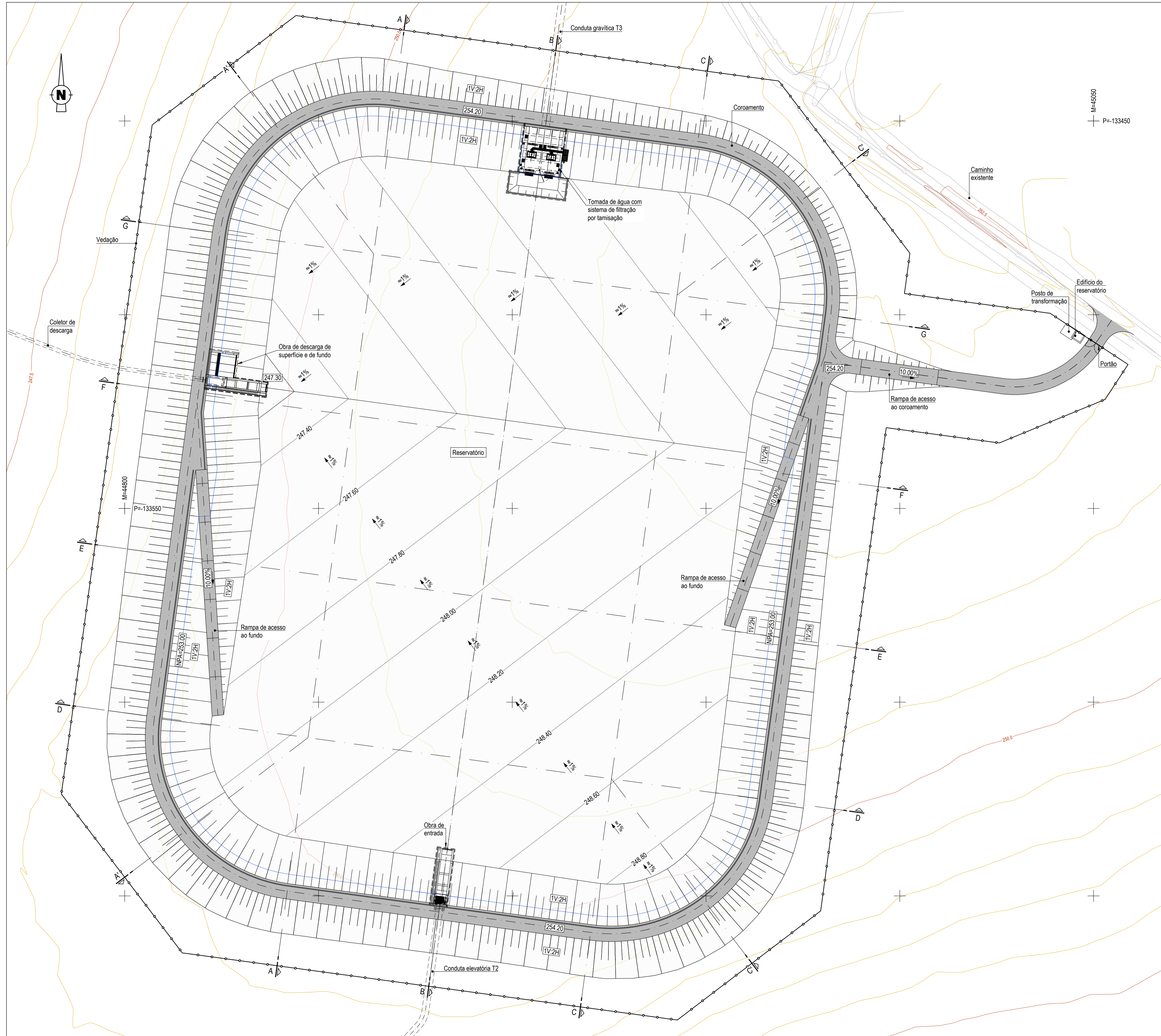
PLANTA Esc. 1:500
