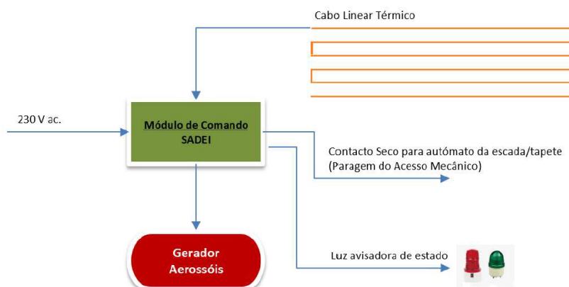
Figura 32 – Sistema SADEI em escadas rolantes
