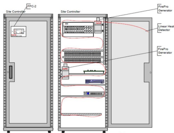
Figura 31 – Sistema SADEI em quadro elétrico
