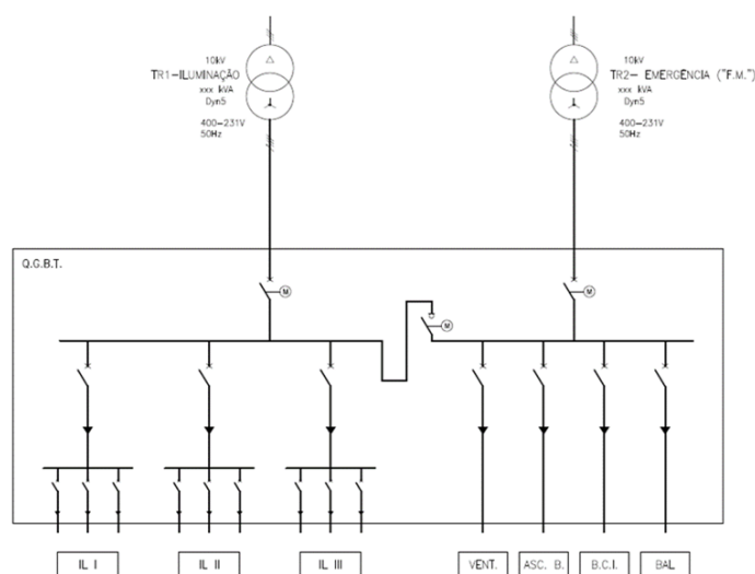
Figura 18: Diagrama tipo da rede de Baixa Tensão
