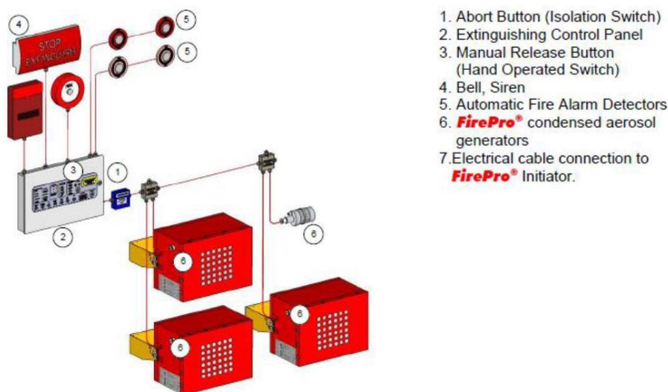
Figura 30 – Diagrama do SADEI em espaços técnicos (INUNDAÇÃO TOTAL)
