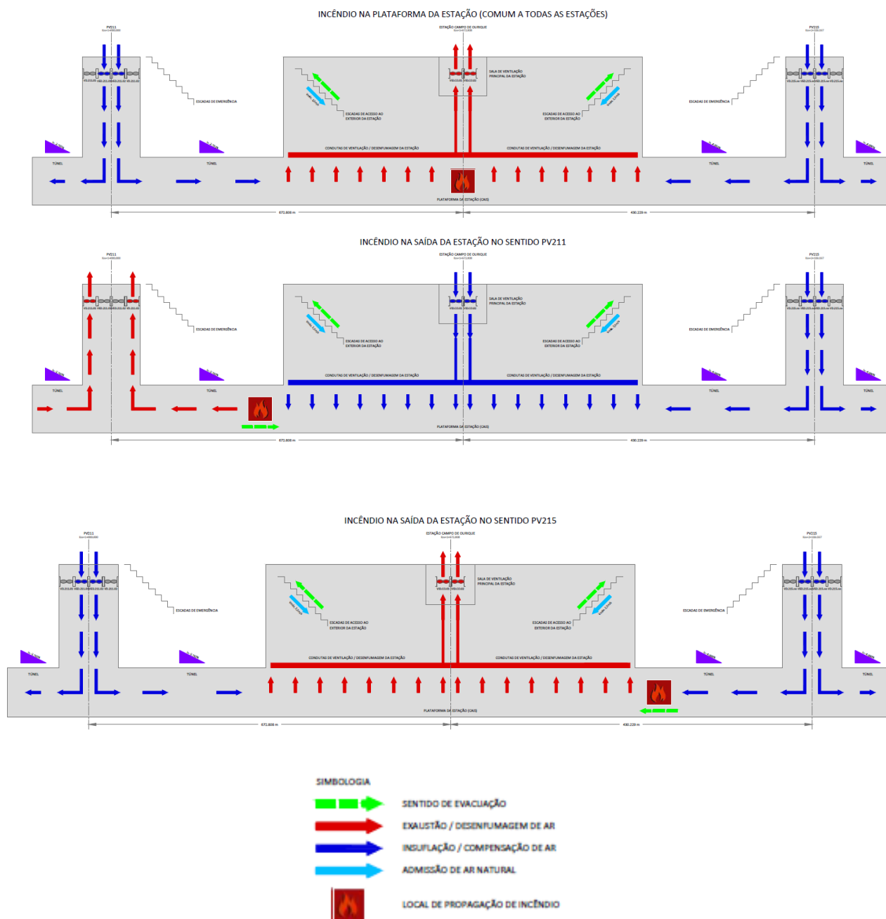
Figura 25 – Cenários de incêndio – Estação Campo de Ourique
