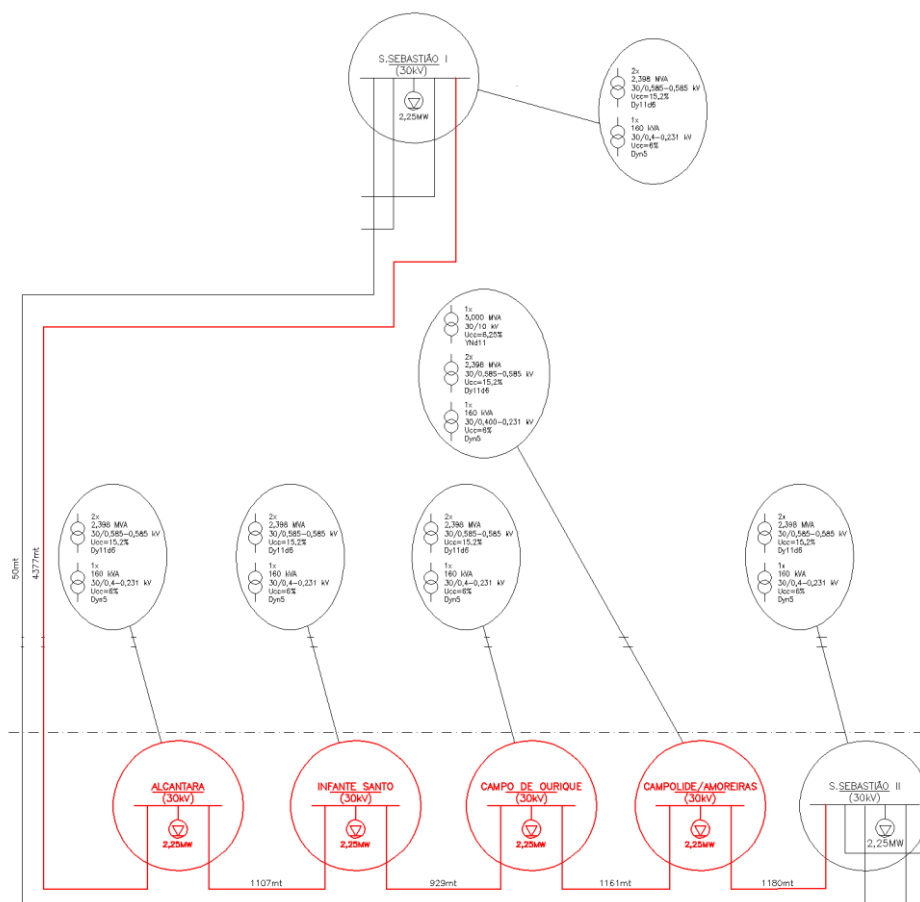
Figura 16: Anel de 30kV da extensão da linha vermelha
