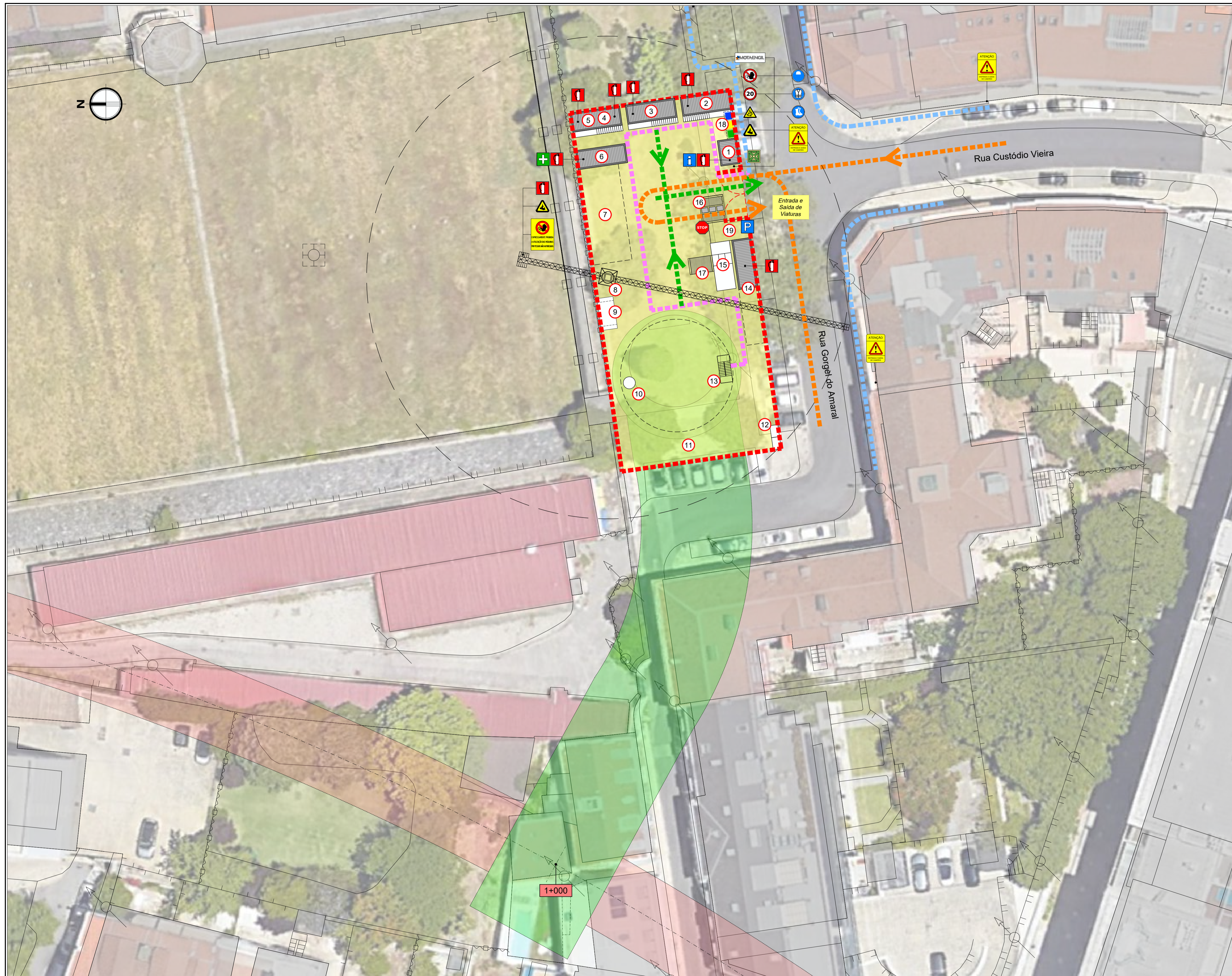
PV211 - Planta de Estaleiro e Sinalização de Segurança A1 - Escala 1:250
