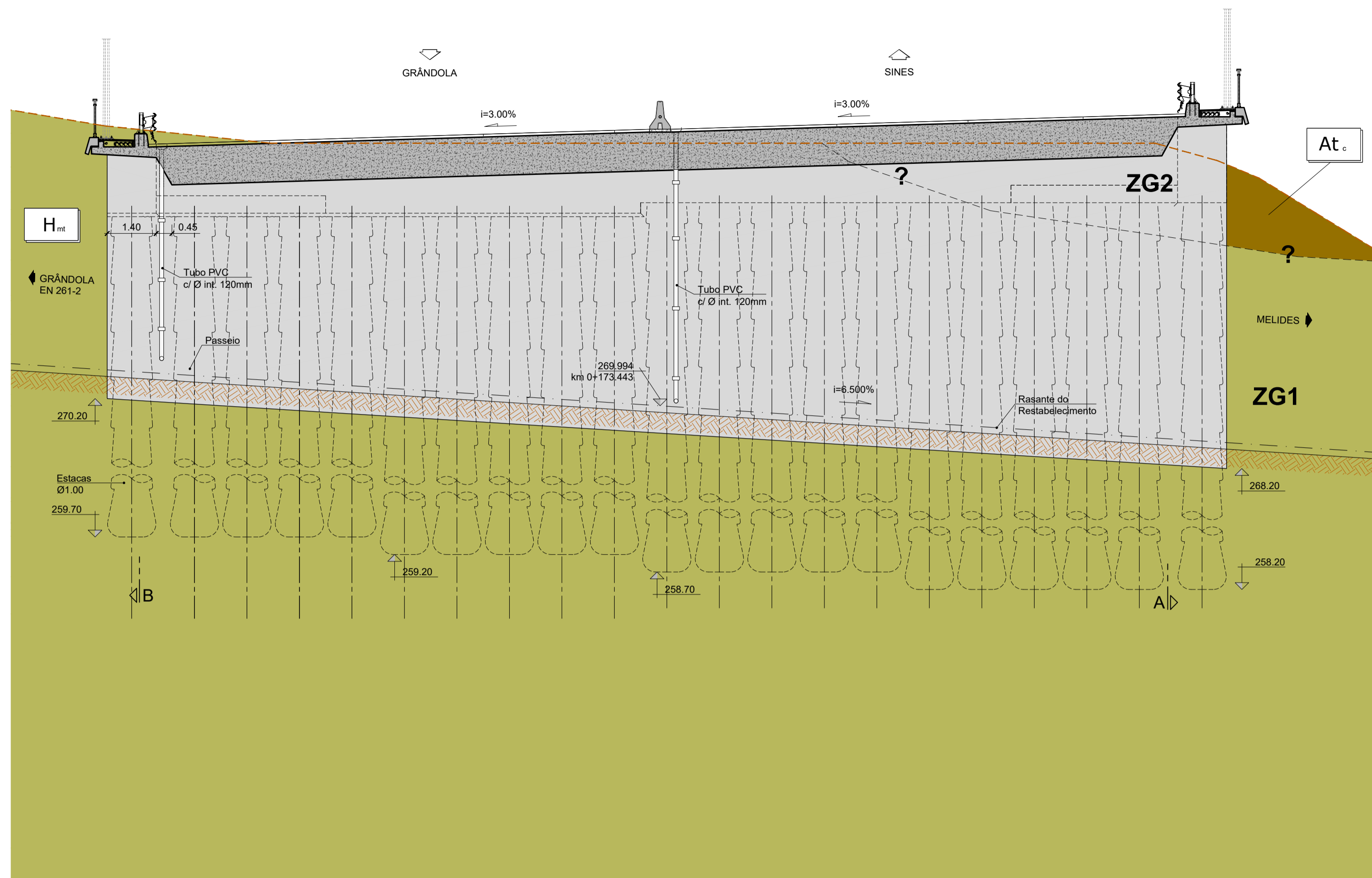
ALÇADO DO ENCONTRO 1 ESC.=1:100
