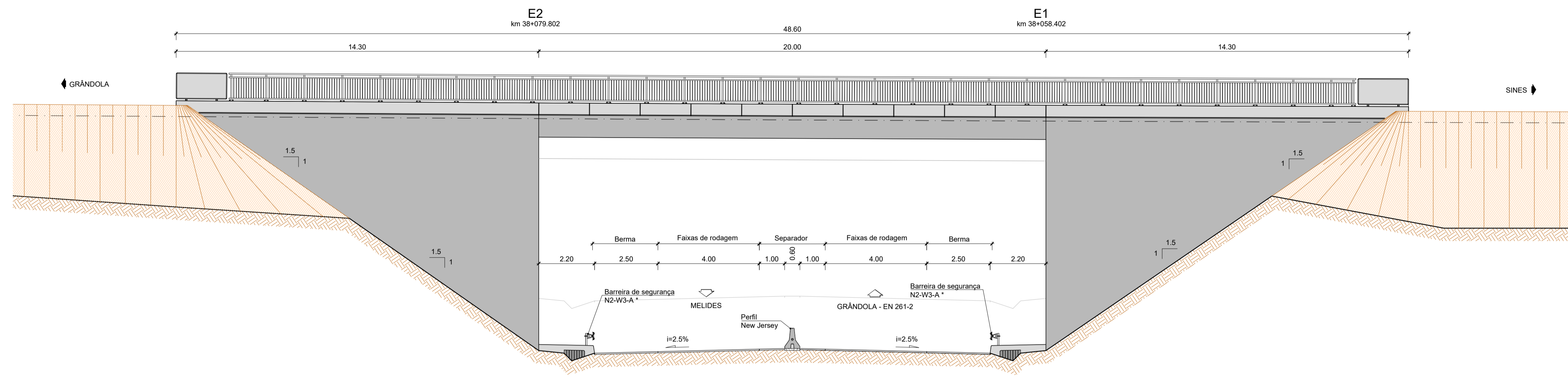
ALÇADO POENTE ESC.=1:100
