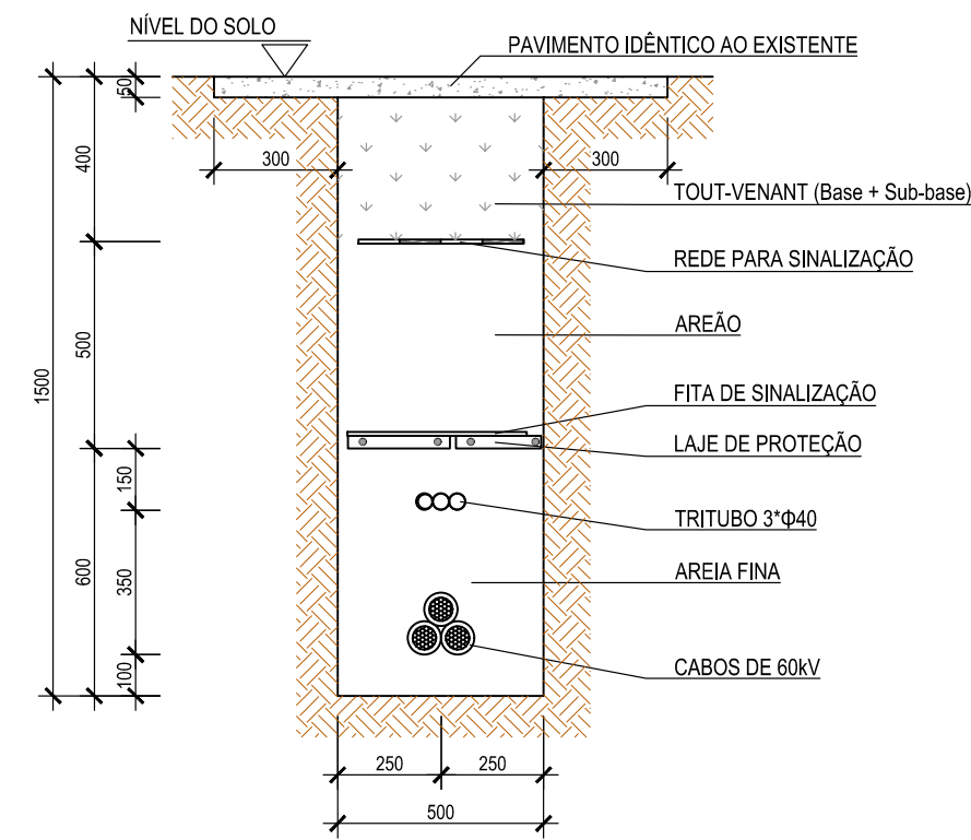
SECÇÃO TIPO VALA S/ ESCALA
