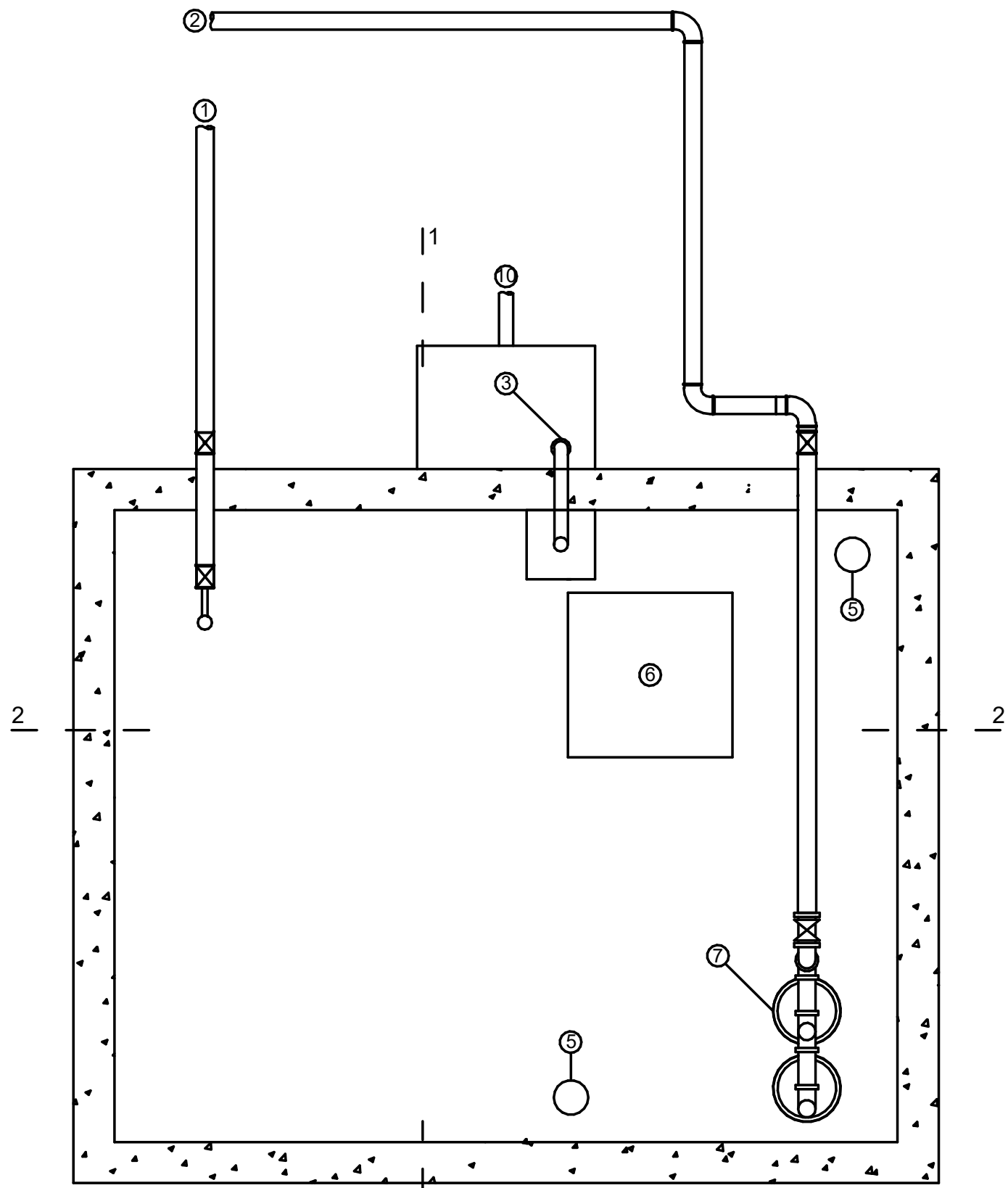
PLANTA/Plant
