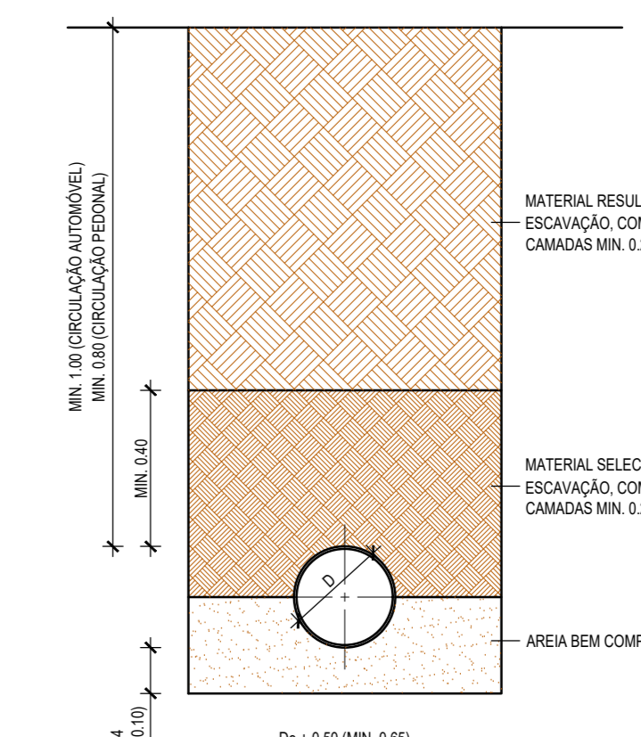
VALAS - CORTE TIPO ESCALA 1:20
