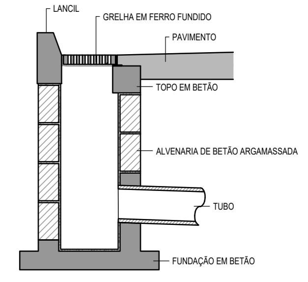
SUMIDOUROS - CORTE ESCALA 1:20
