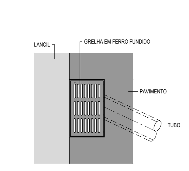
SUMIDOUROS - PLANTA ESCALA 1:20
