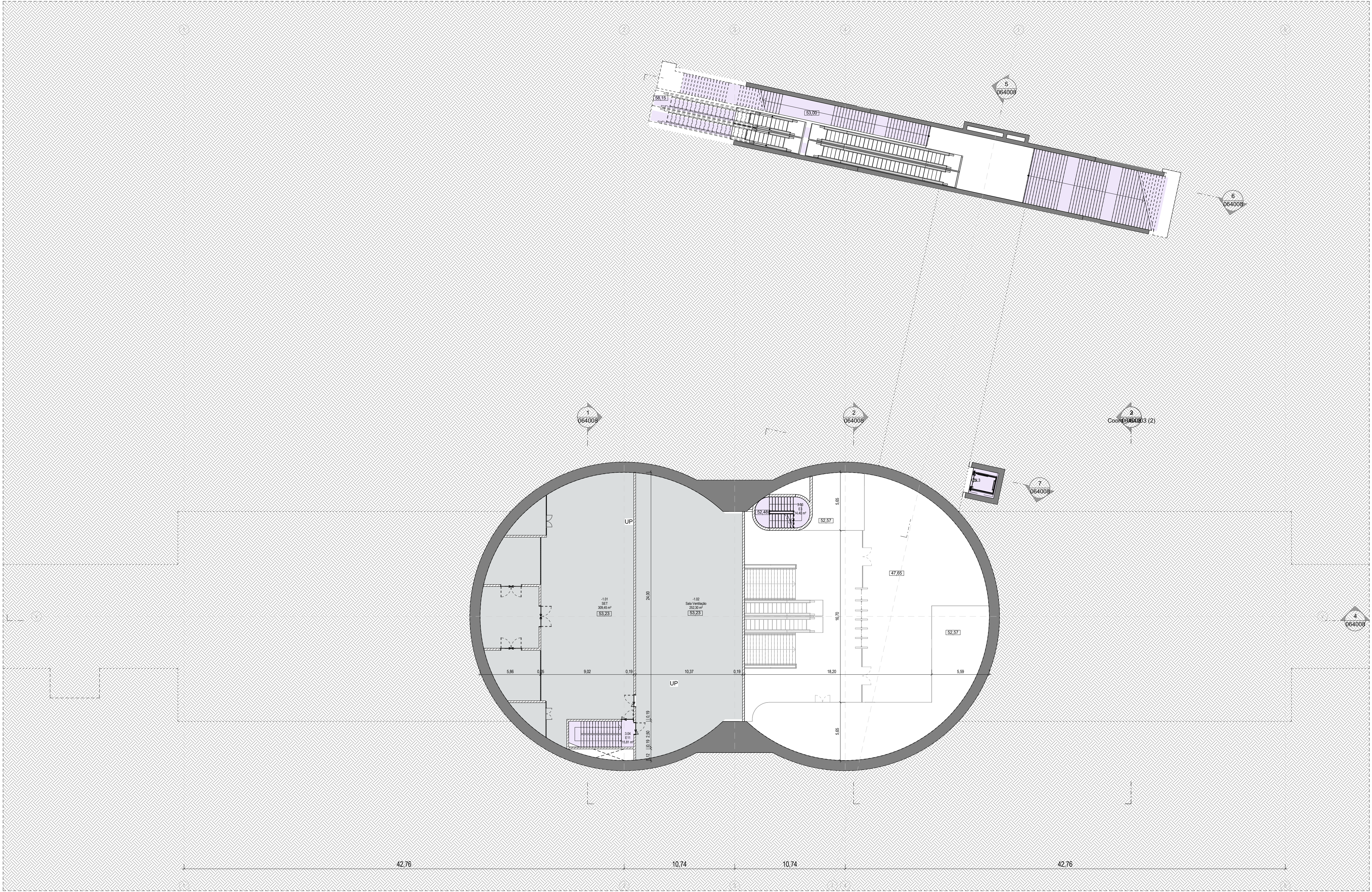
PLANTA DO SET E VENT 1 : 200
