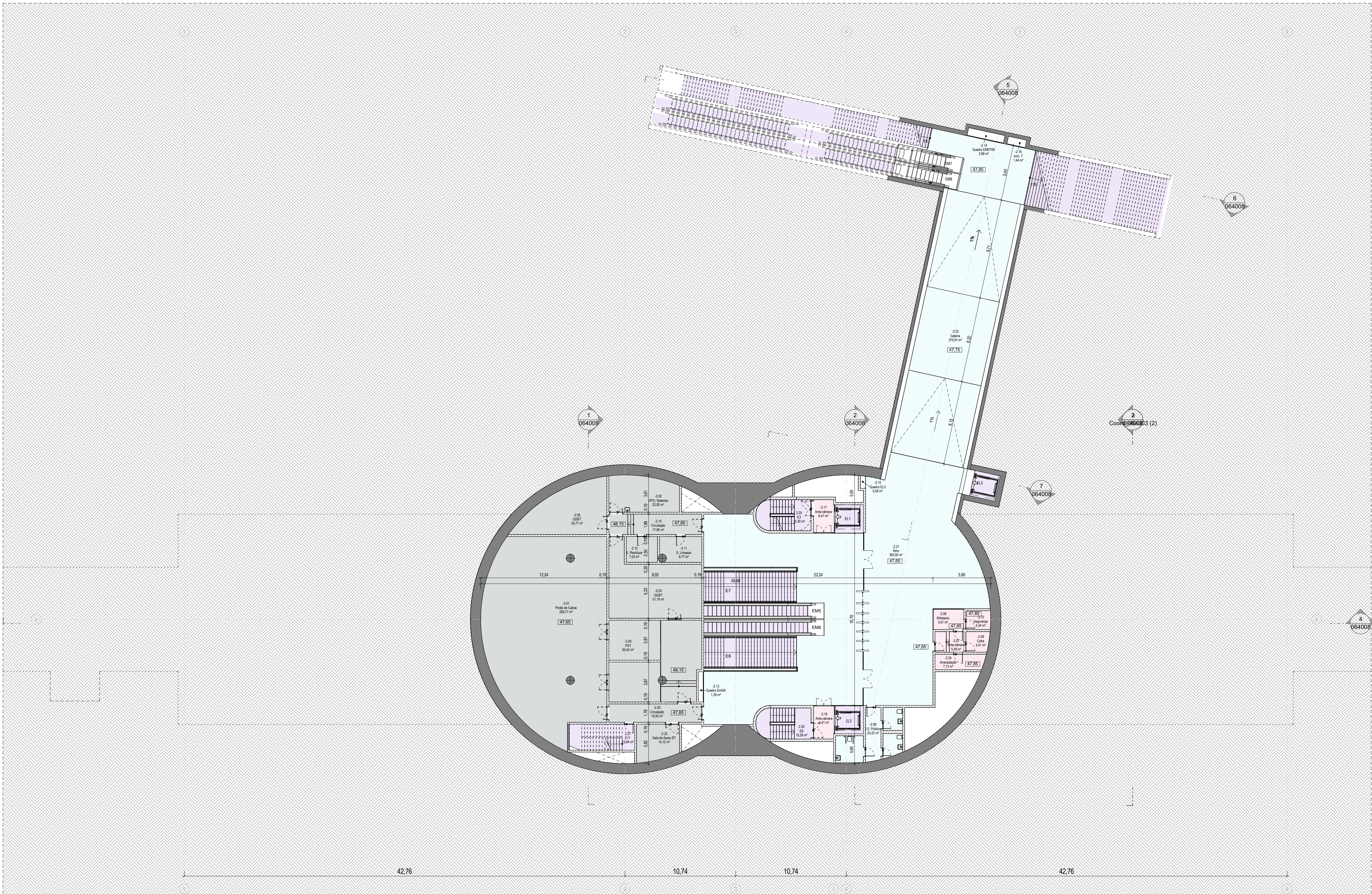
PLANTA DO ÁTRIO 1 : 200
