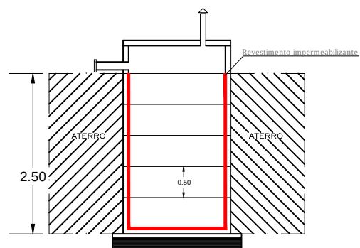
CORTE C-D
