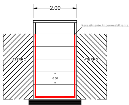
CORTE A-B
