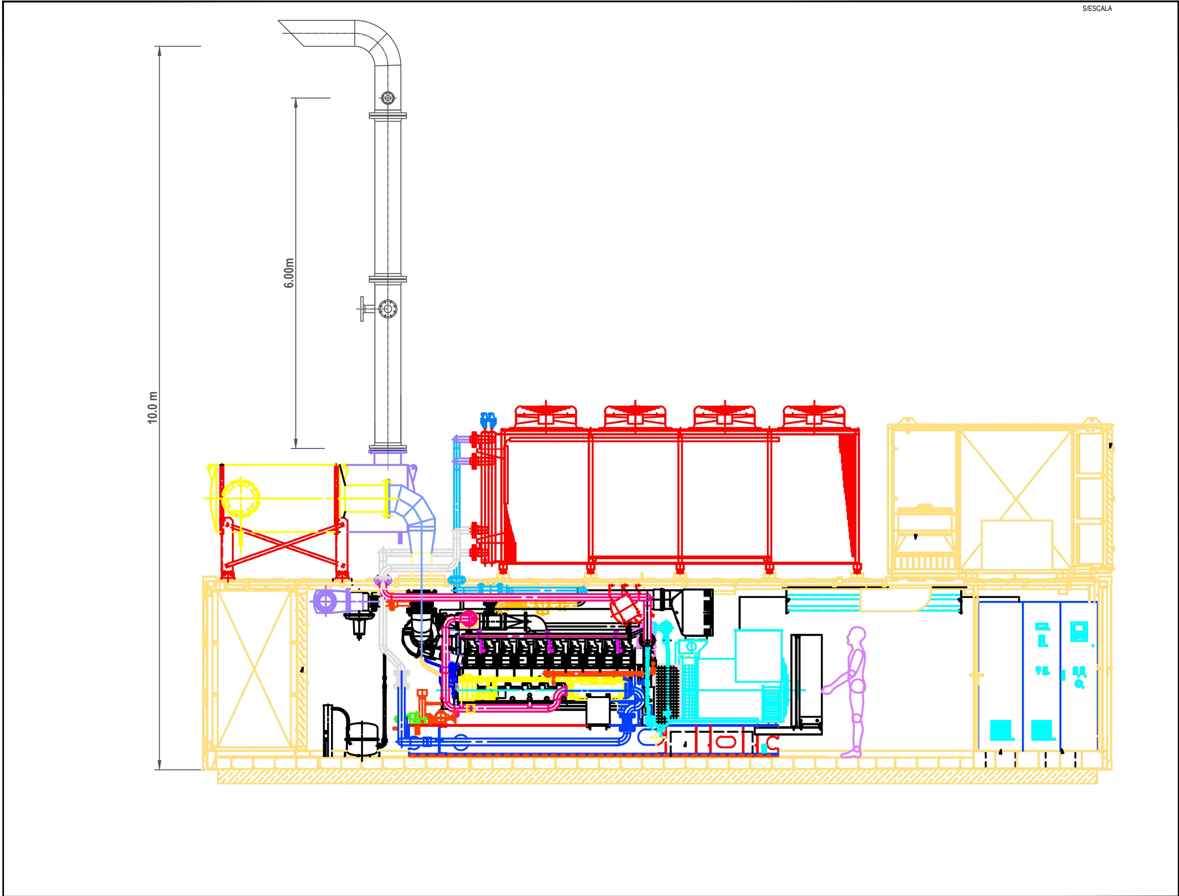
PLANTA DE ENQUADRAMENTO
