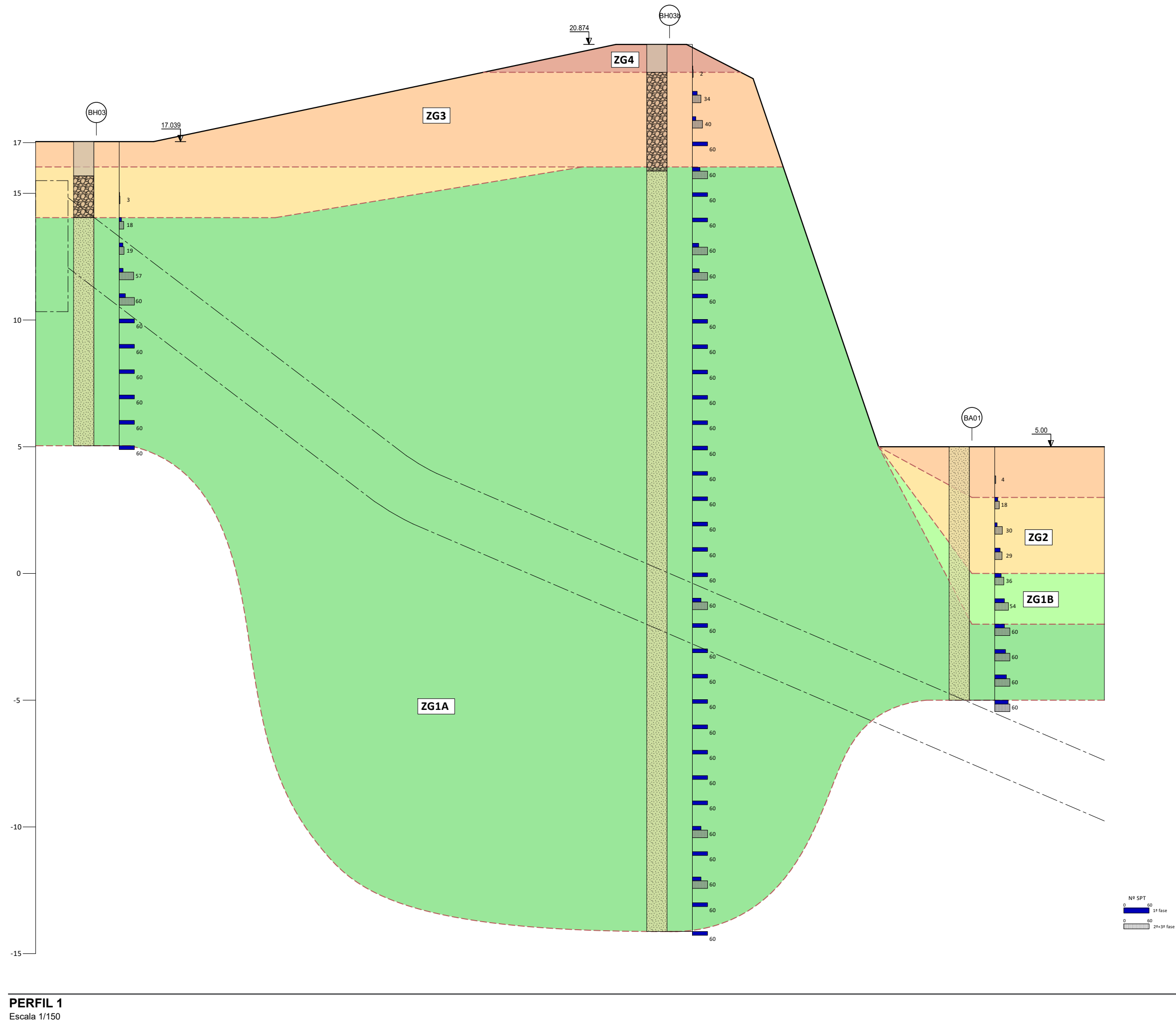
PERFIL 1 Escala 1/150
