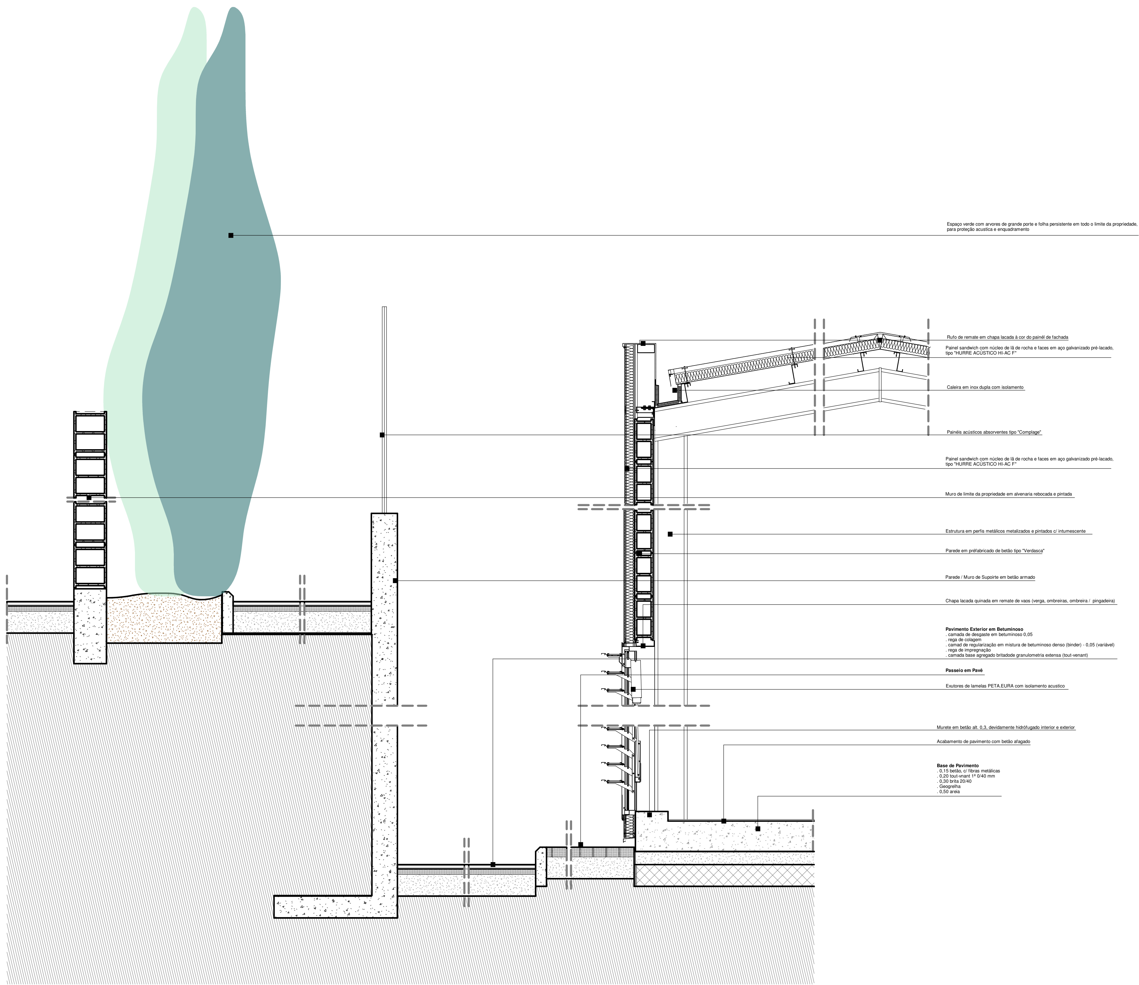
Pormenor Construtivo Tipo 1 : 20
