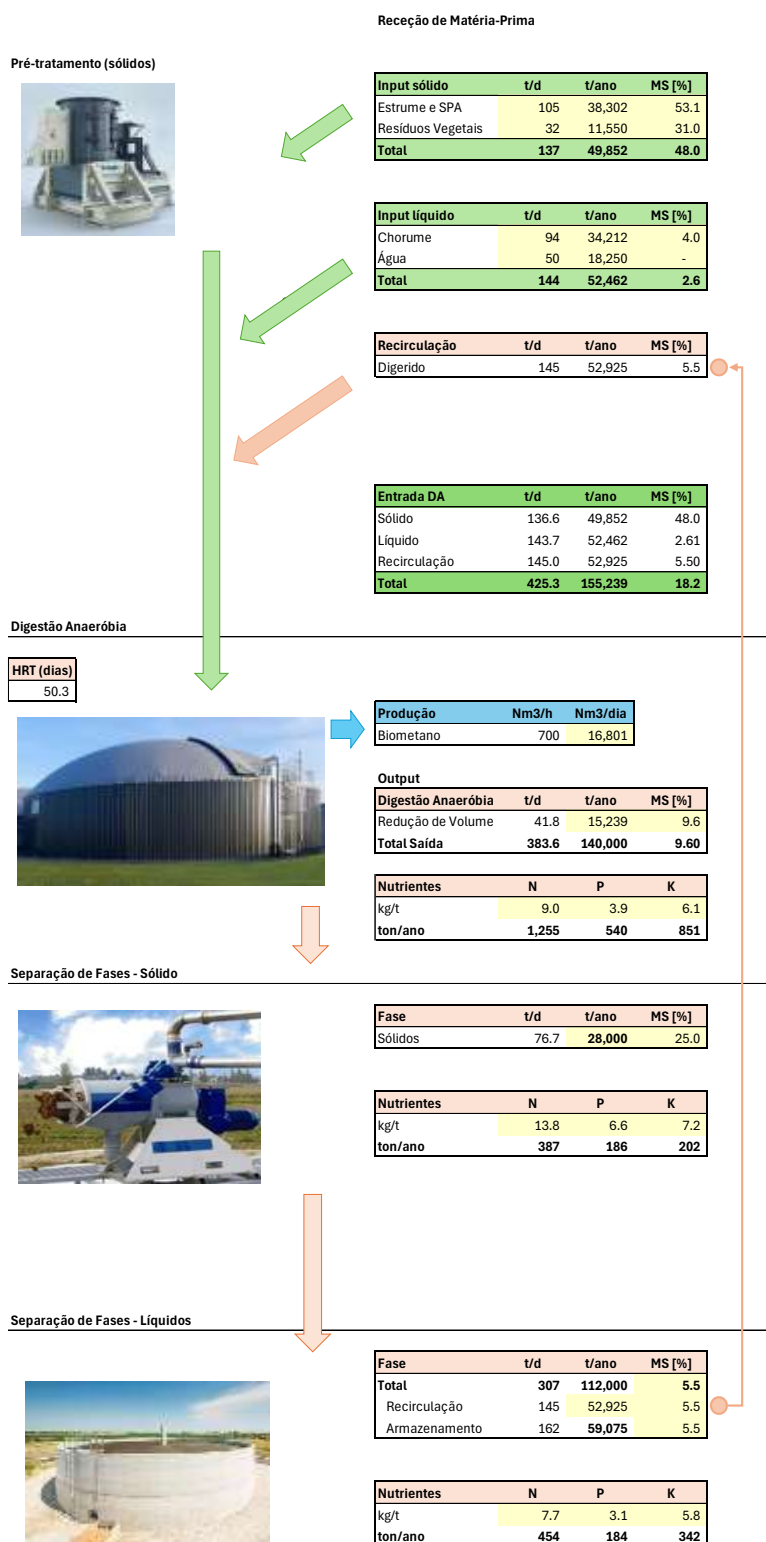
Figura 4.6 – Balanço de Massas completo - UB Abrigada
