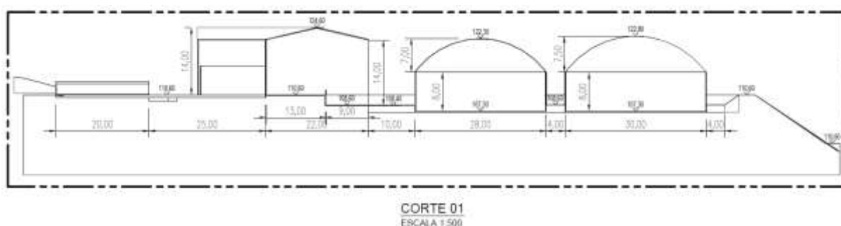
Figura 4.4 – Corte na Zona de Retenção e Digestores
