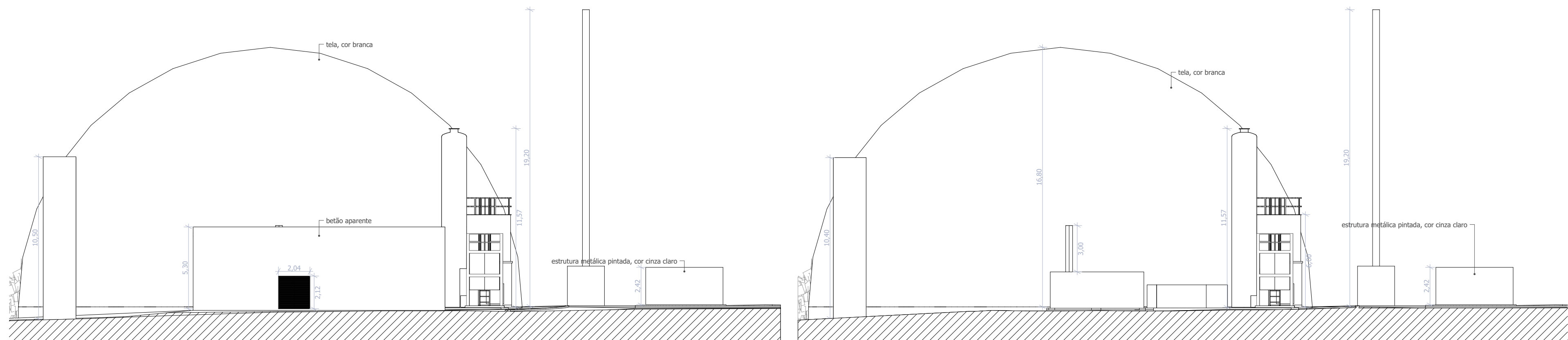
alçado A.05.B
