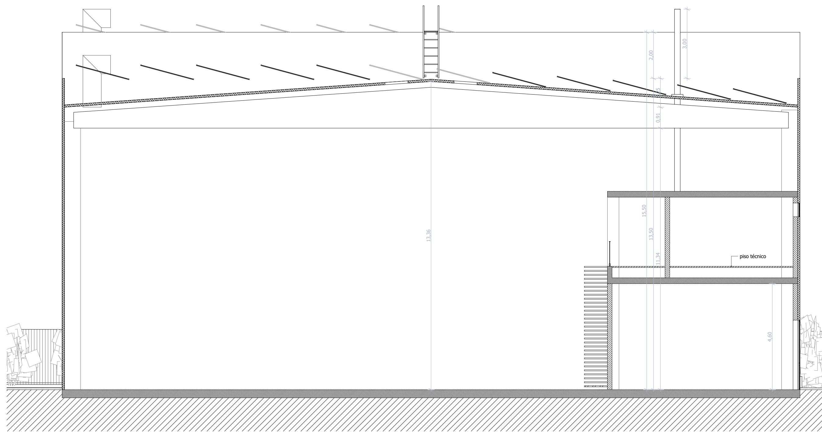
Corte C.03.C
