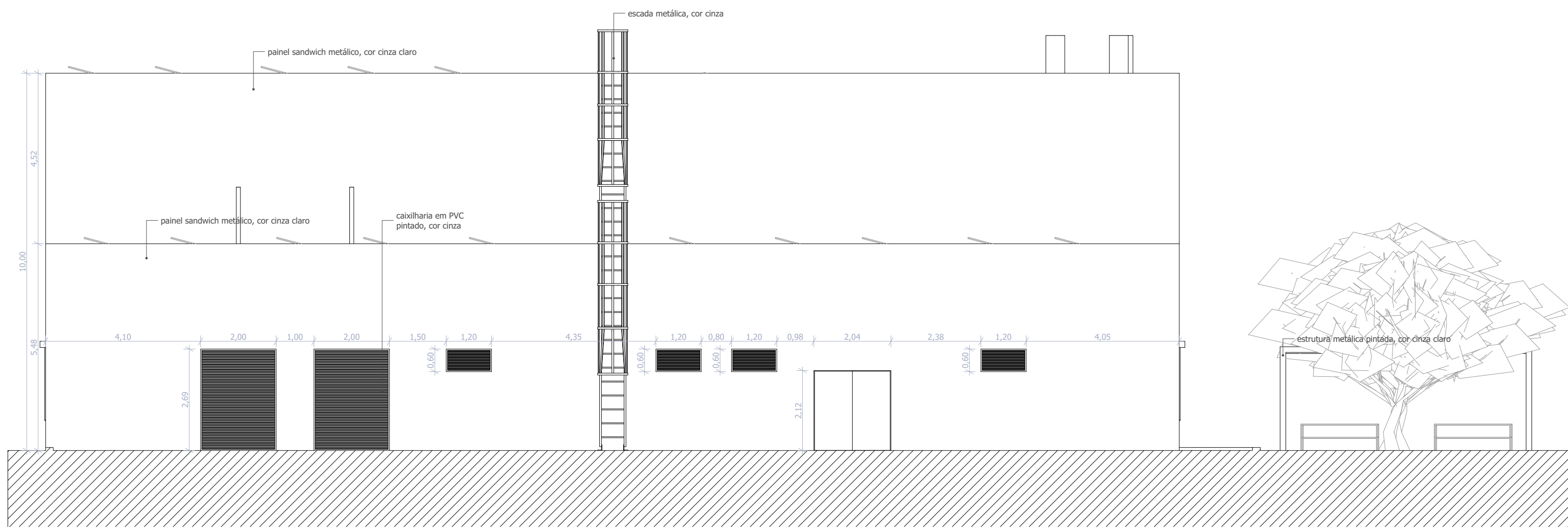
alçado A.02.D
