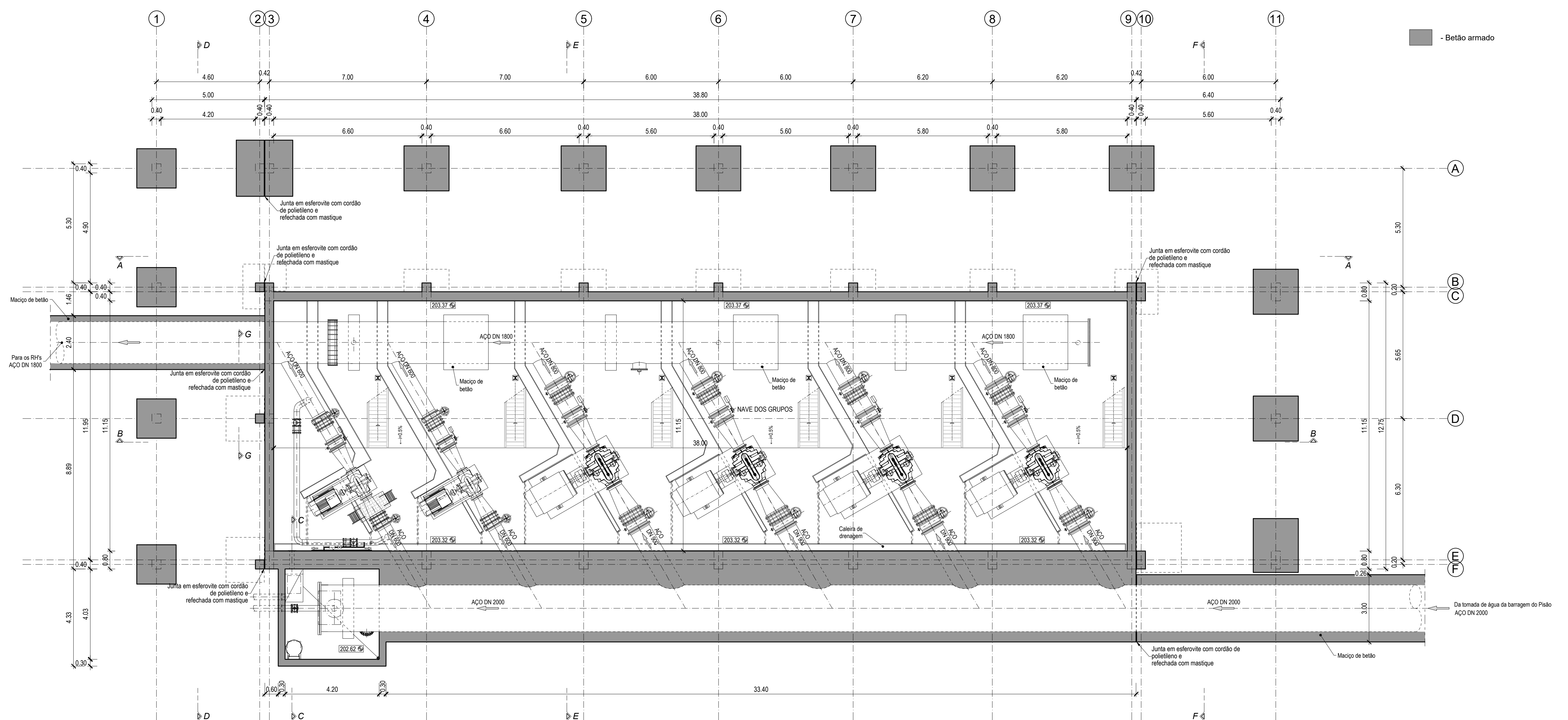
PLANTA (Cota 204.90) Escala 1:100
