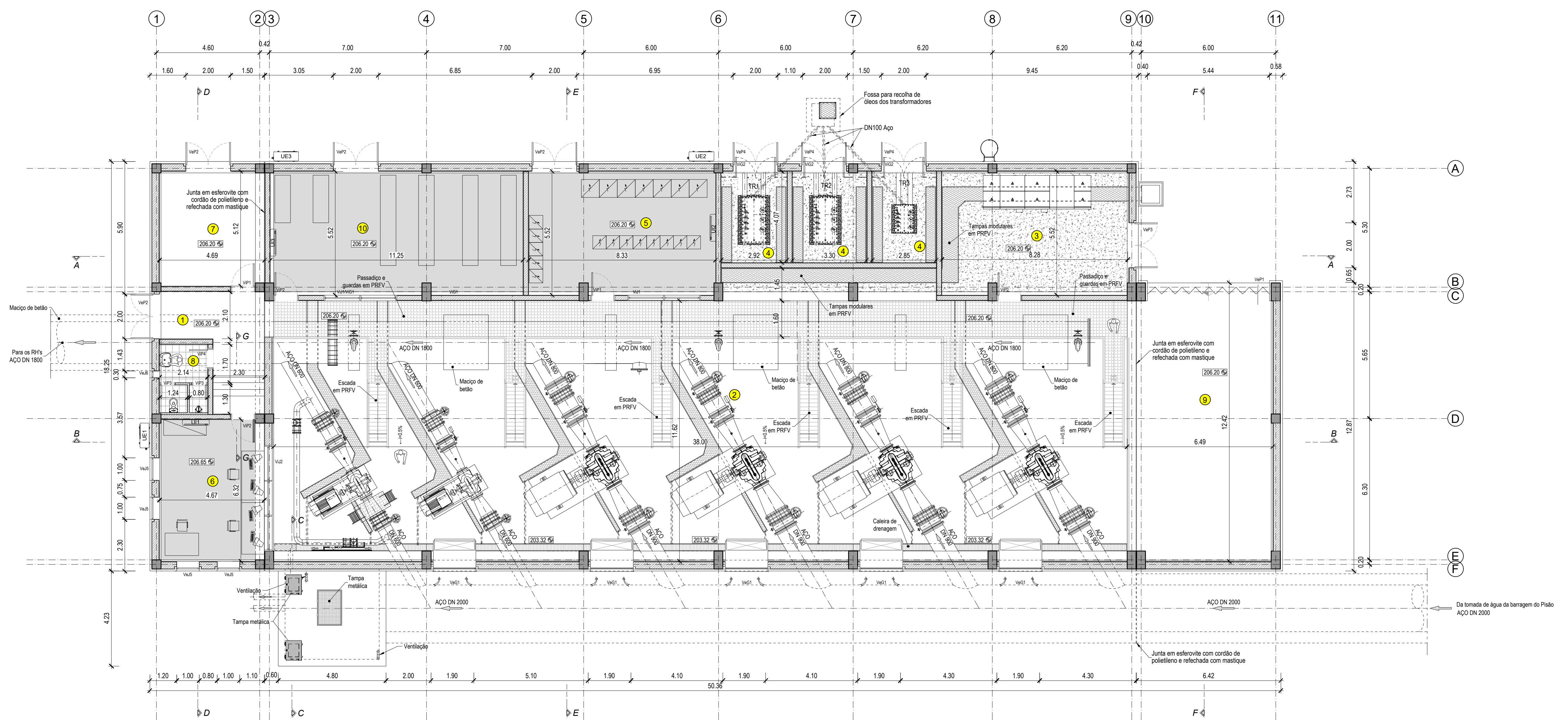
PLANTA GERAL Escala 1:100
