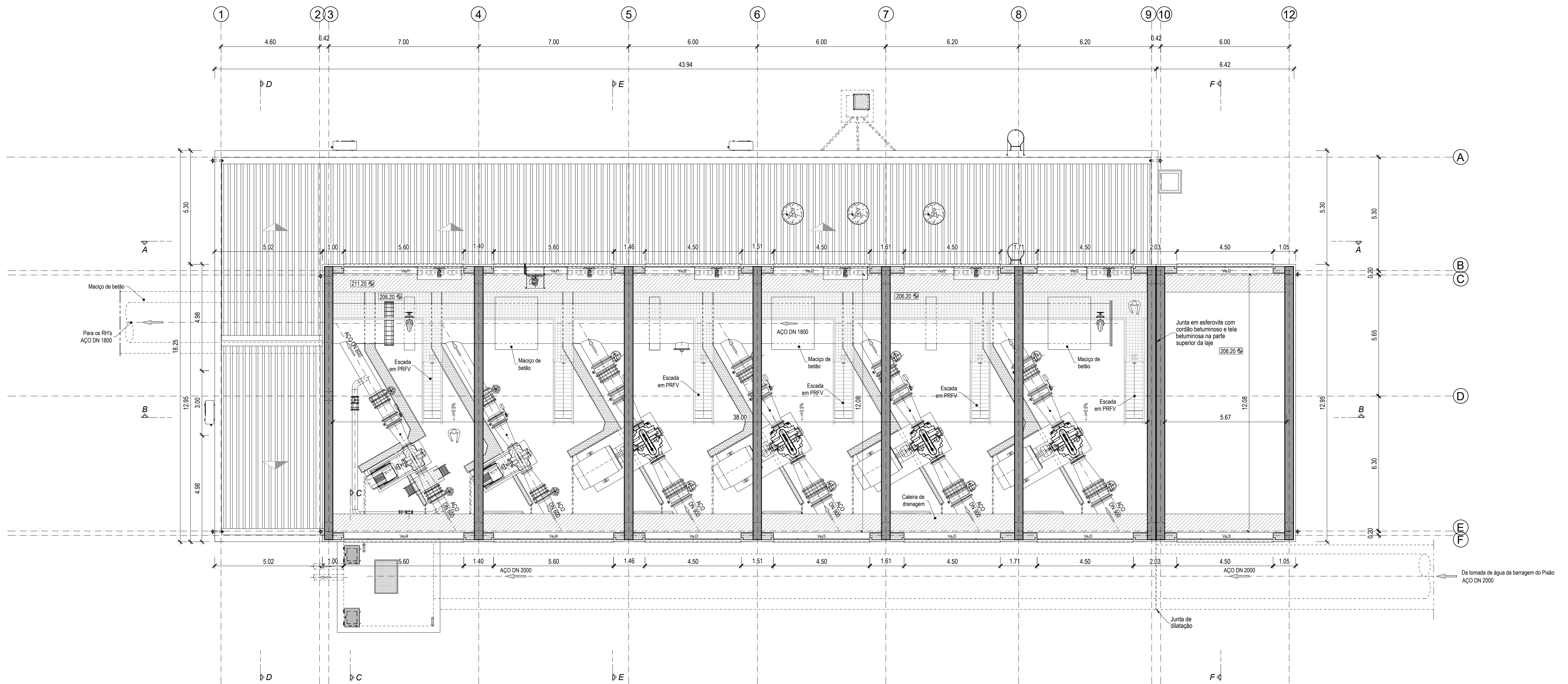
PLANTA (Cota 212.50) Escala 1:100
