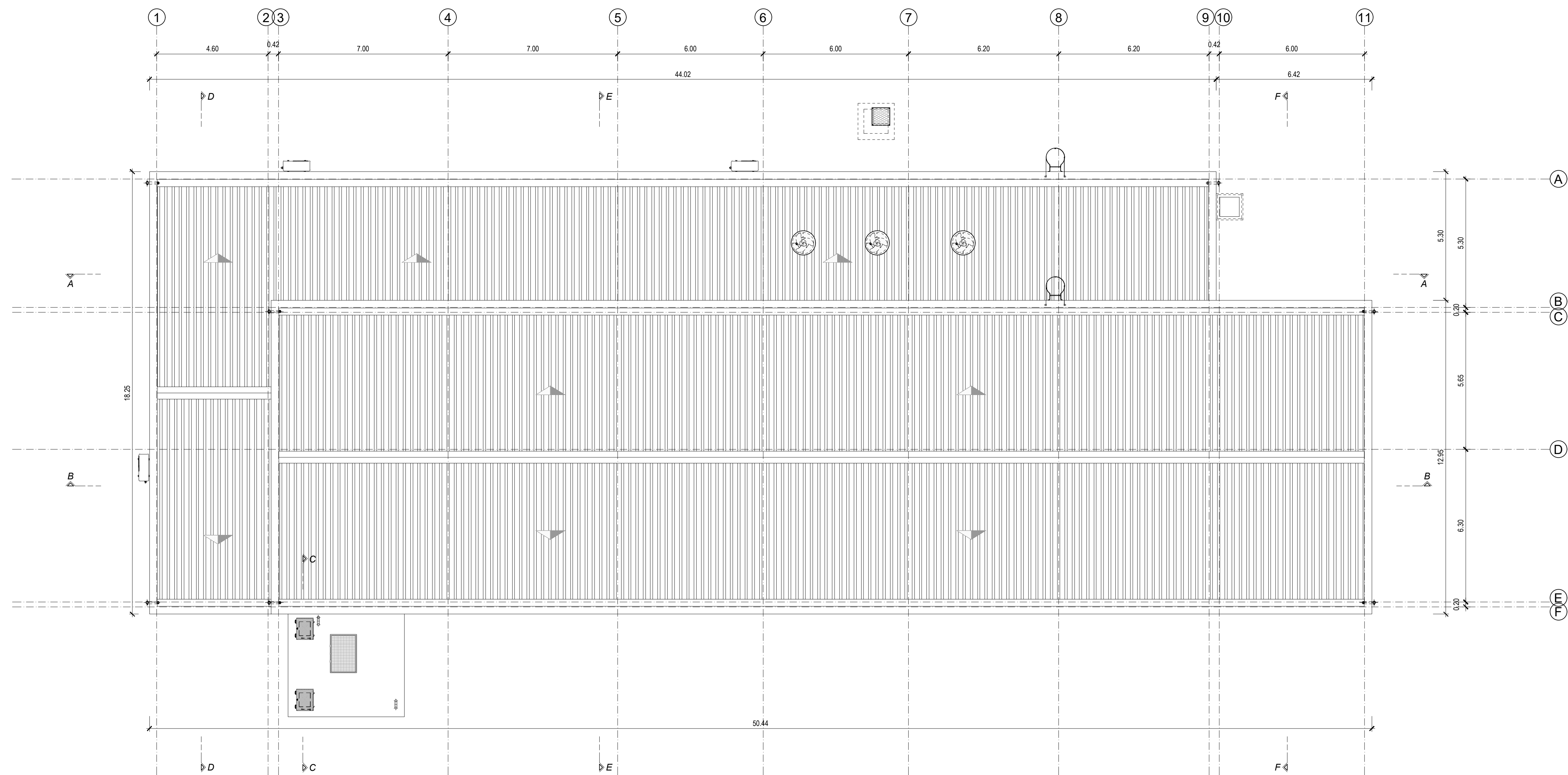
PLANTA DE COBERTURA Escala 1:100
