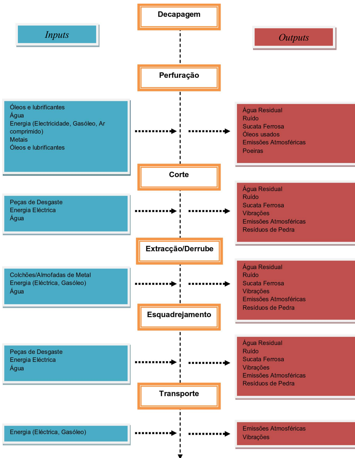
Layout de processo extractivo, com indicação de inputs e outputs .
