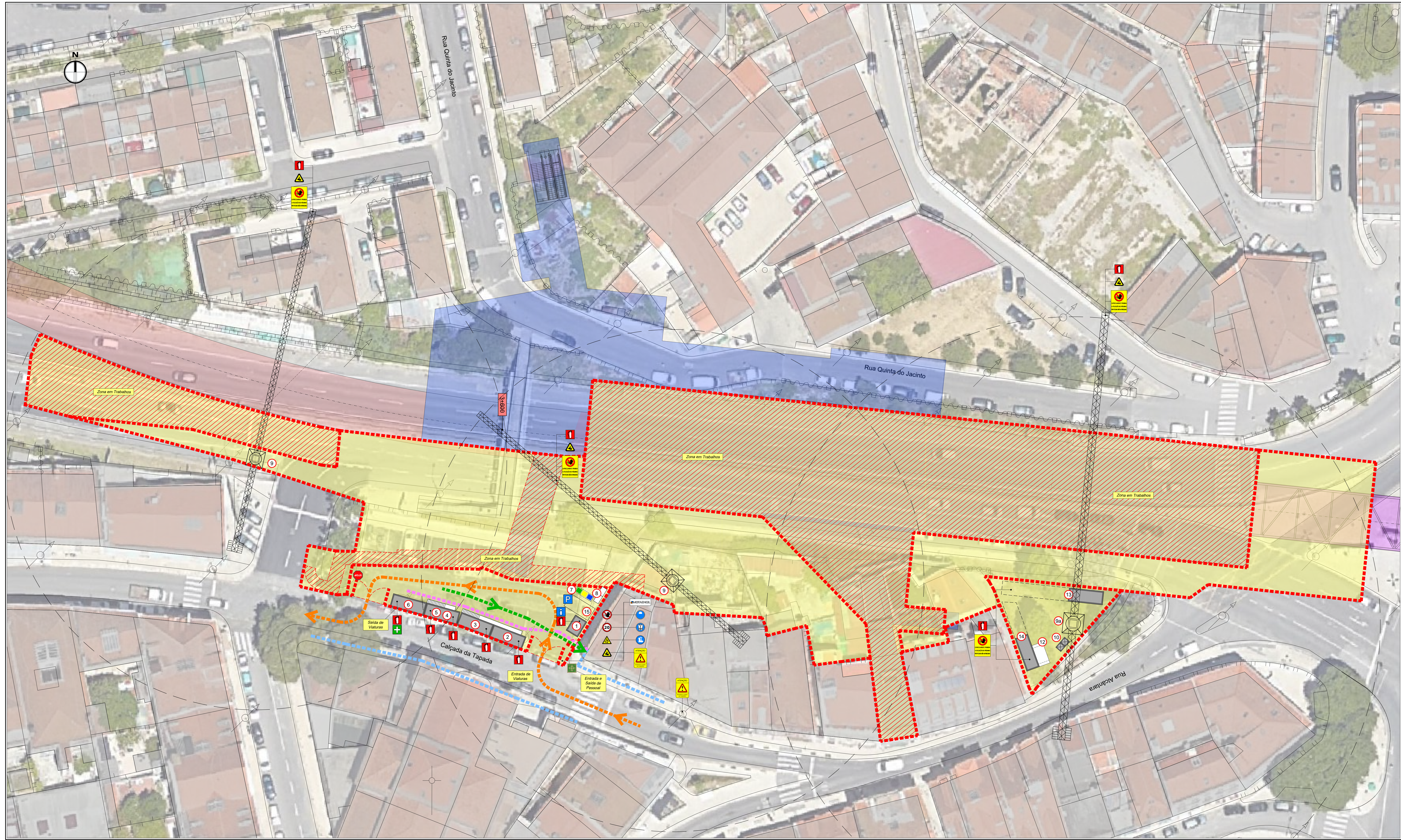
Estação Alcântara - Planta de Estaleiro e Sinalização de Segurança - Fase 3 A0 - Escala 1:200
