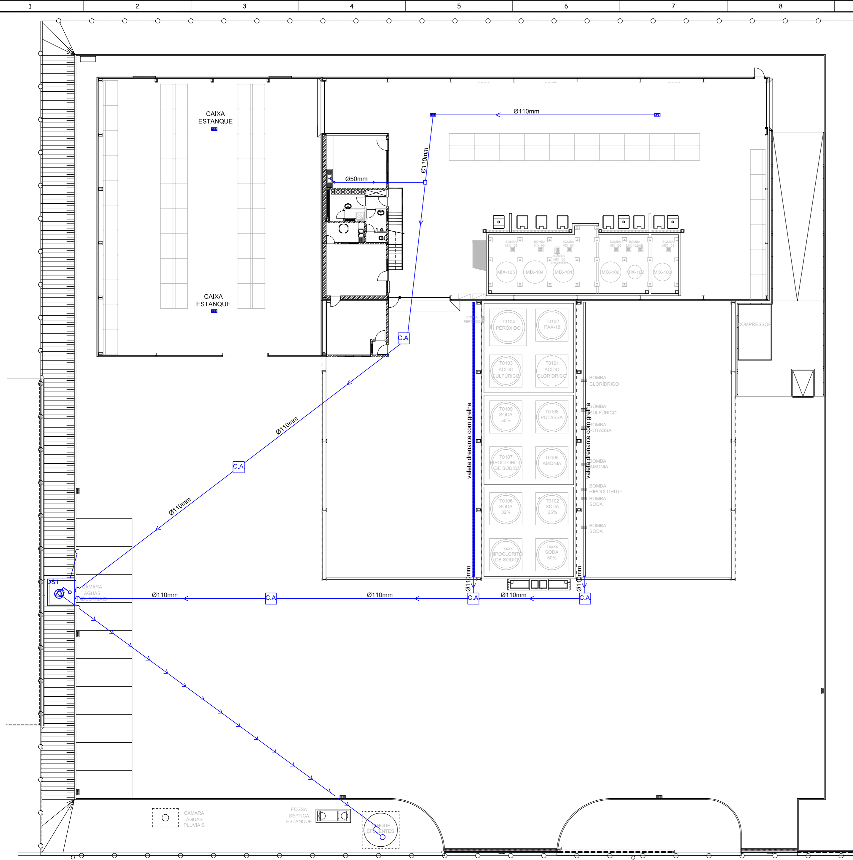
PLANTA ESCALA: 1/200
