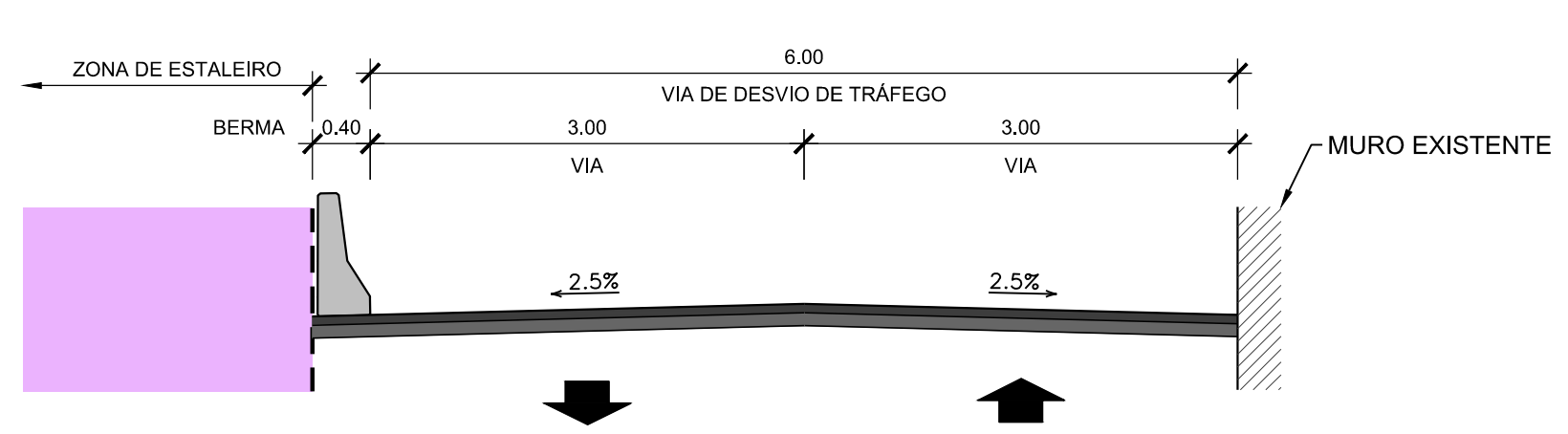
SECÇÃO A-A' ESC. 1:50
