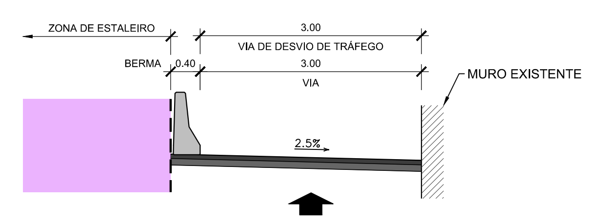
SECÇÃO B-B' ESC. 1:50
