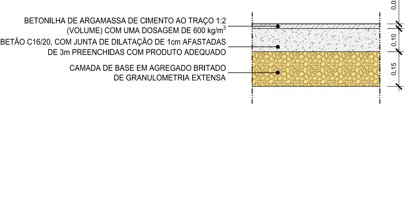
PAVIMENTO PROVISÓRIO DE CIRCULAÇÃO PEDONAL ESC. 1:10
