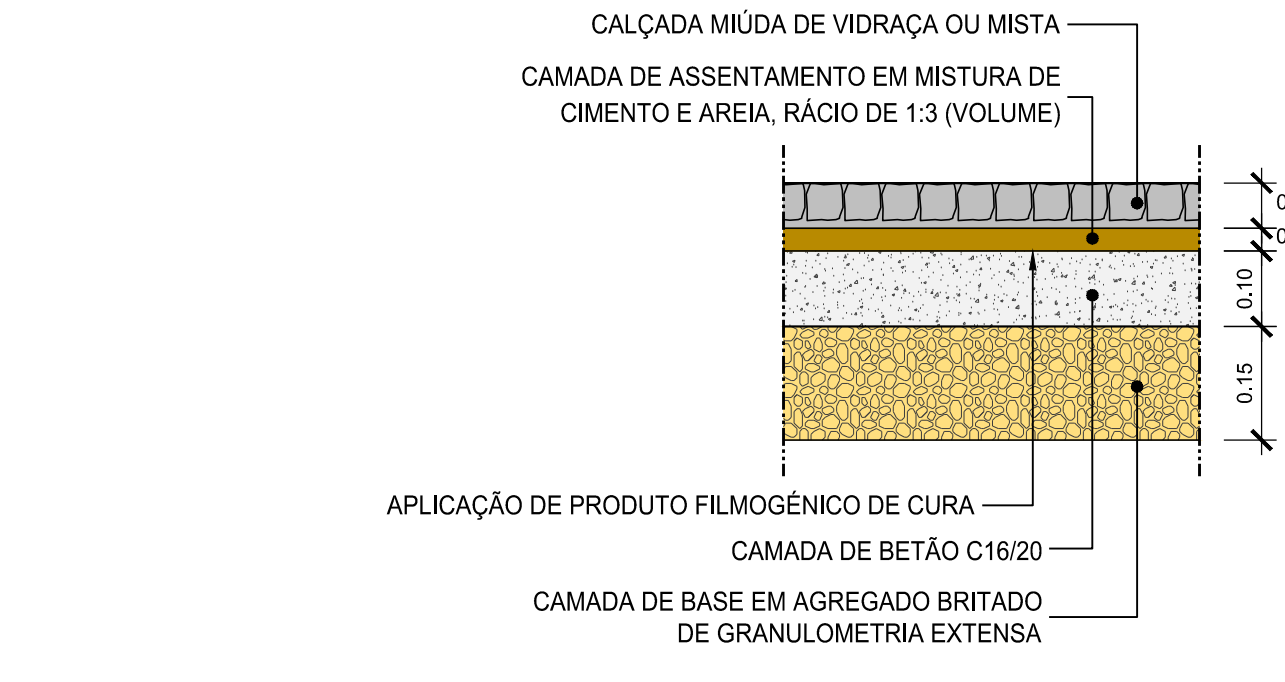
PAVIMENTO DEFINITIVO DE CIRCULAÇÃO PEDONAL ESC. 1:10
