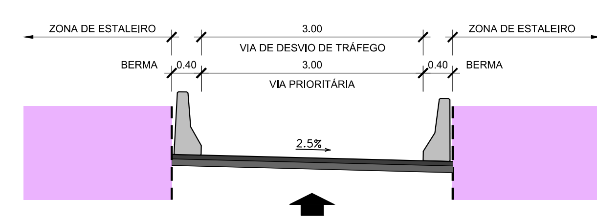
SECÇÃO C-C' ESC. 1:50
