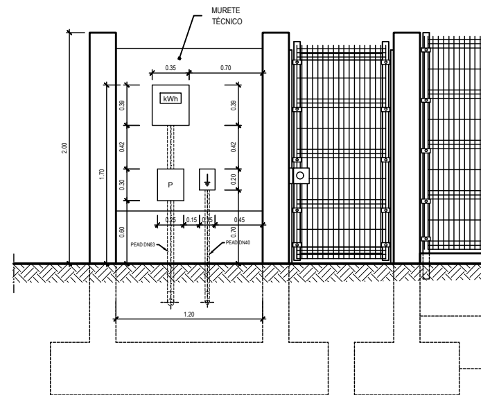
MURETE TÉCNICO A Construir Junto da Entrada
