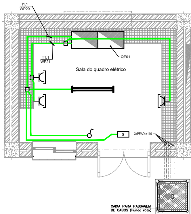
ILUMINAÇÃO E TOMADAS INTERIOR
