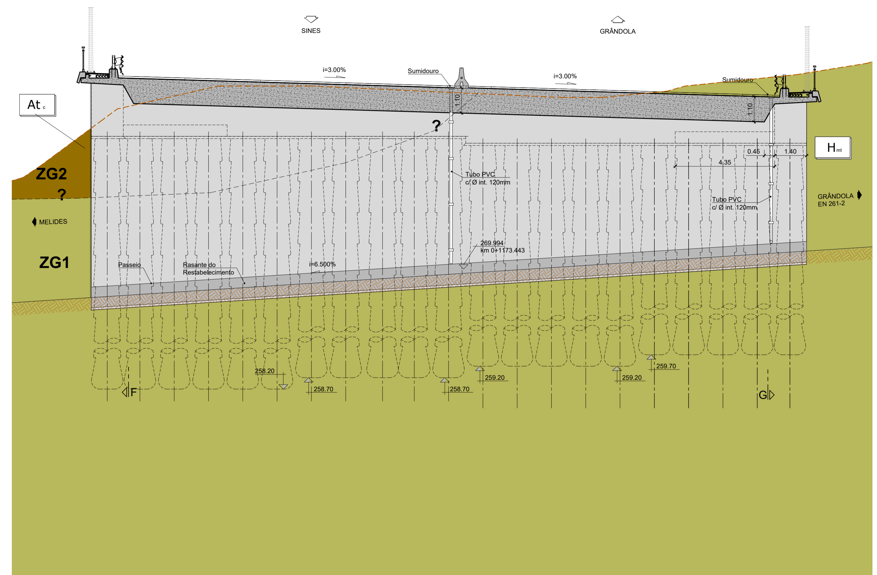
ALÇADO DO ENCONTRO 2 ESC.=1:100
