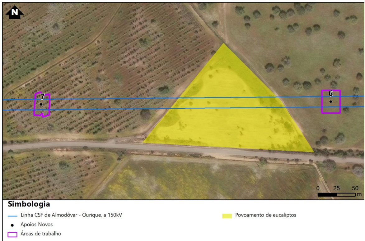
Figura 2.1 – Povoamento de eucalipto sobrepassado pelo vão 6-7 da linha
