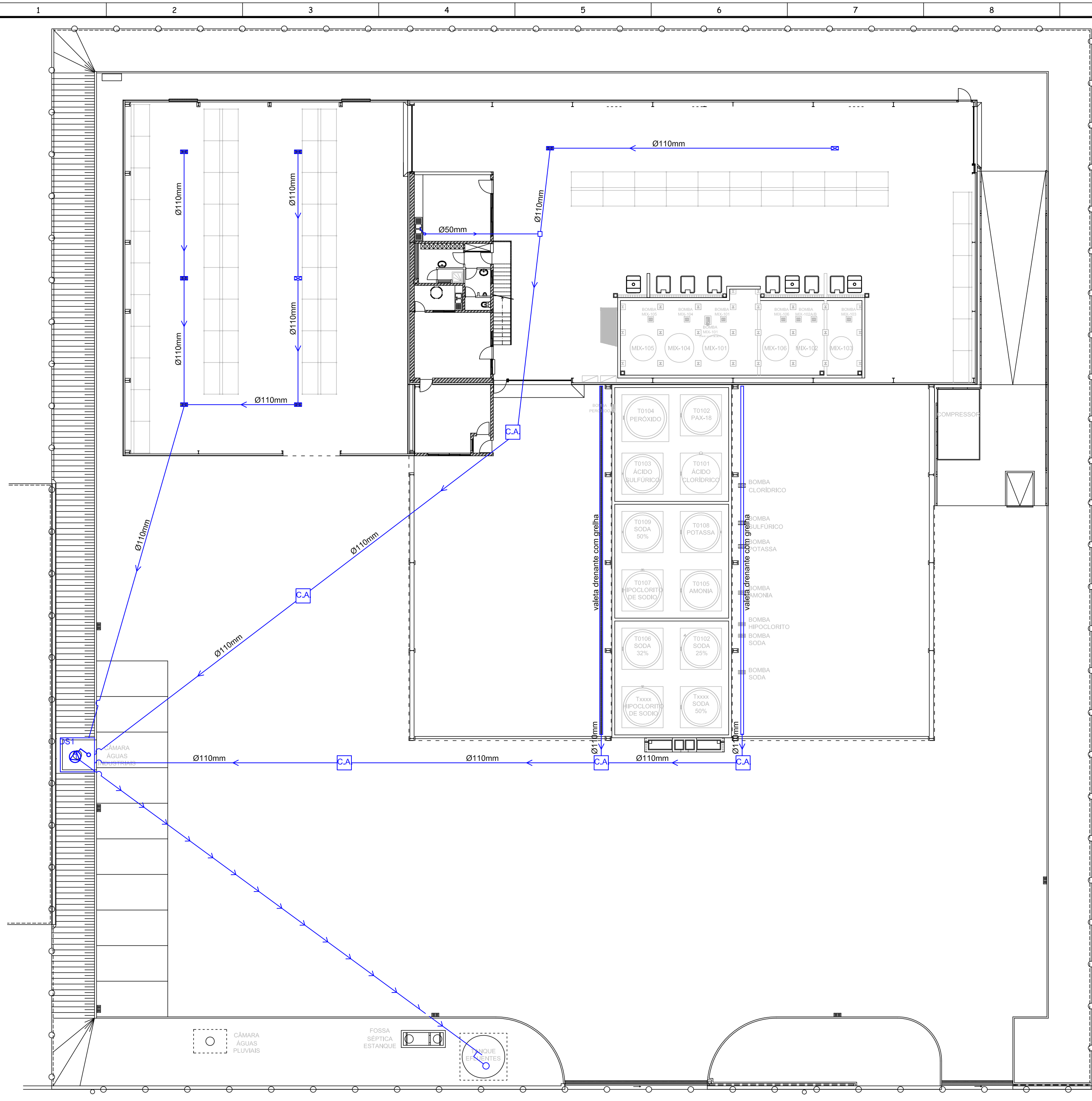
PLANTA ESCALA: 1/200
