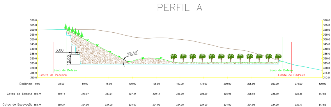
Figura 2 - Ângulo de talude durante a fase de enchimento
