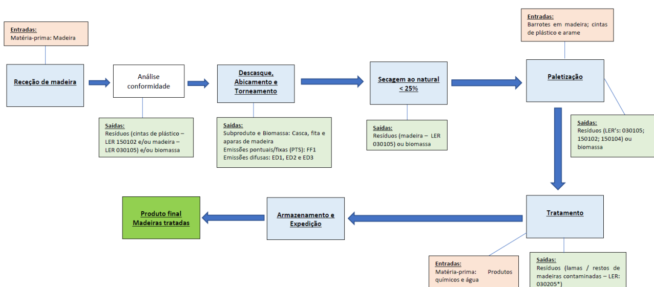
Figura 1 - Processo Produtivo de Madeiras Tratadas (Impregnação de Madeira)
