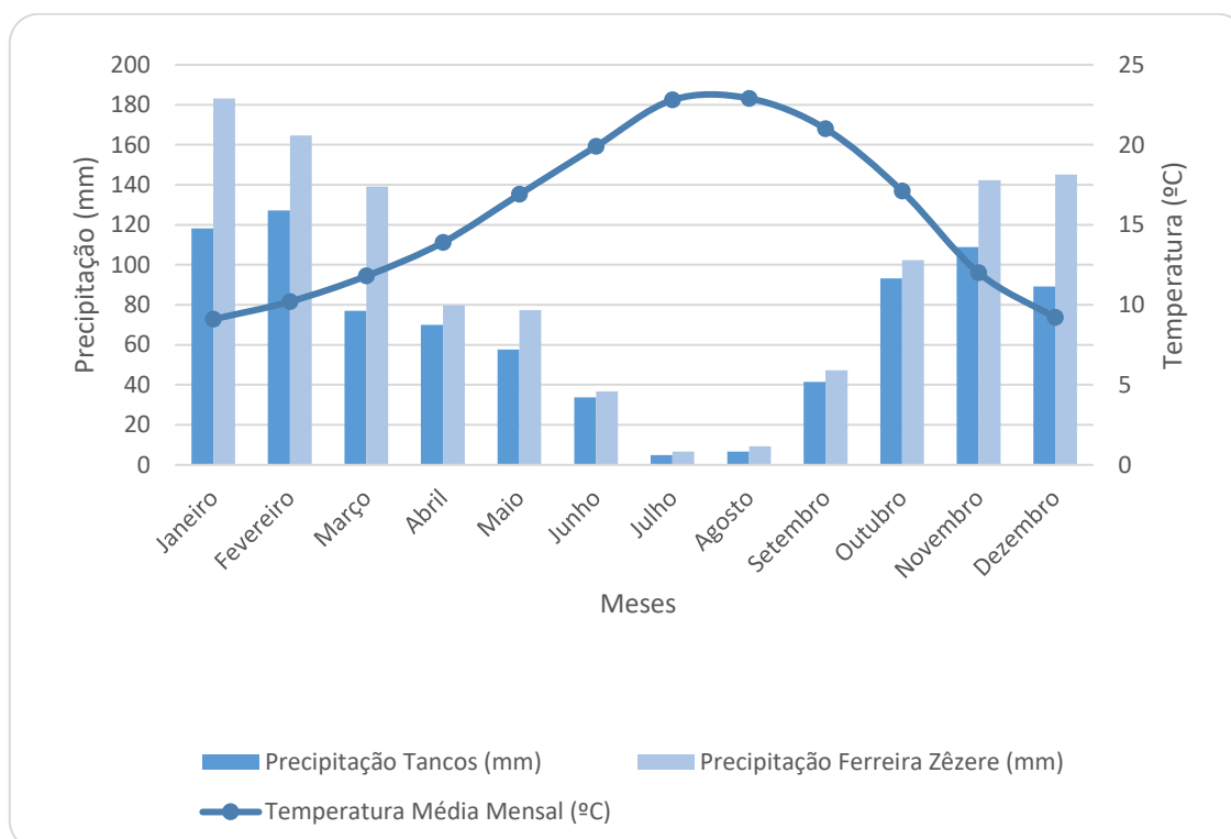
Figura 7.3 - Gráfico Termo-pluviométrico nas estações climatológicas de Tancos/ Base Aérea e udométrica de Ferreira do Zêzere (1951-1980)
