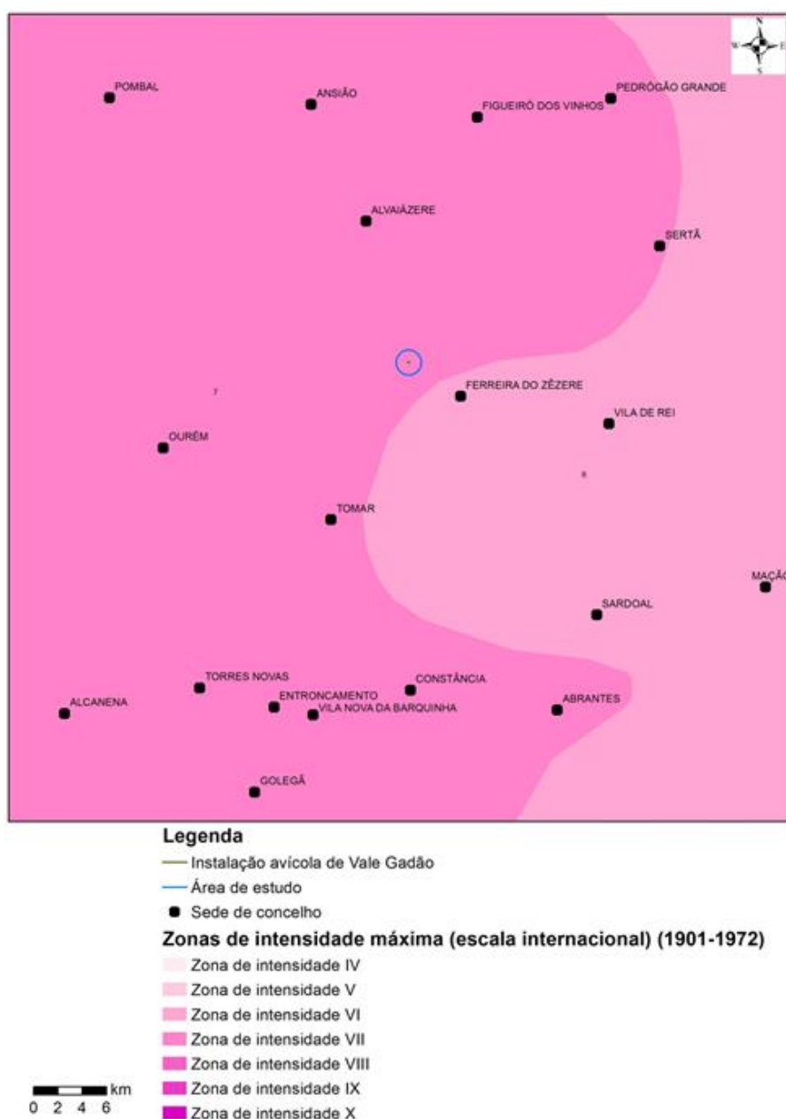
Figura 7.12 – Isossistas de intensidades máximas, na escala internacional, para a intensidade sísmica em Portugal Continental no período 1901 – 1972 (adaptado do Atlas do Ambiente).
