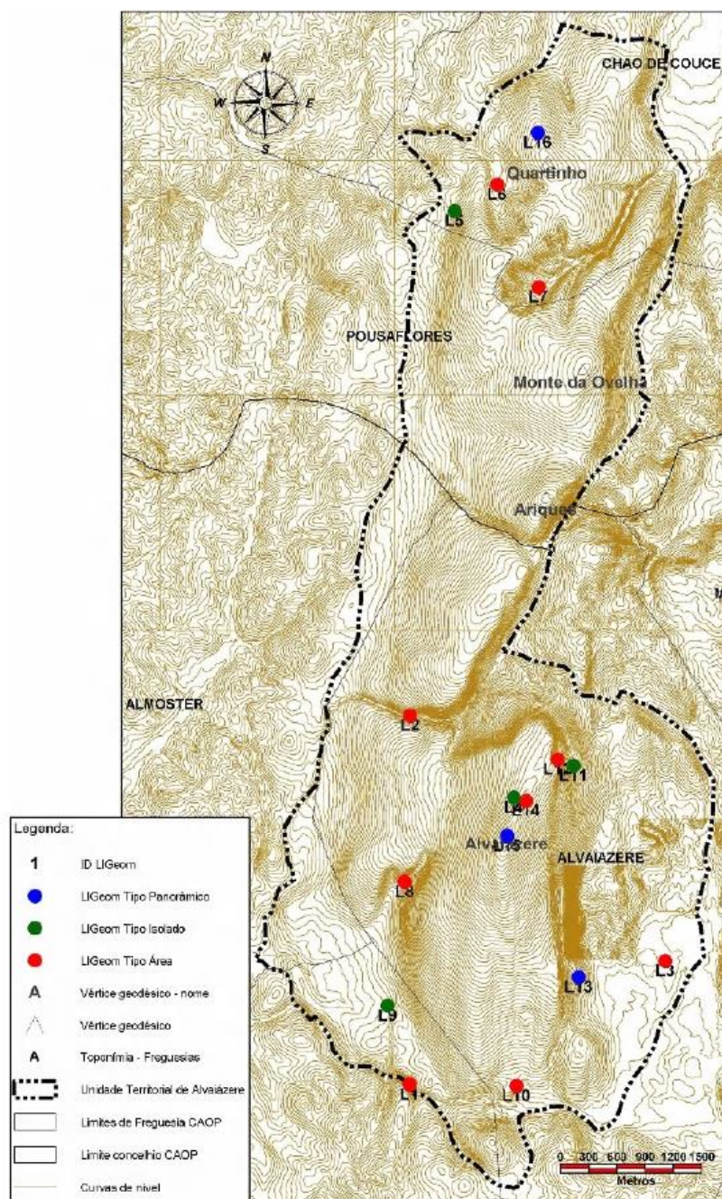
Figura 7.11 - Locais de interesse geológico e geomorfológico na área cársica dos concelhos de Ansião e Alvaiázere (retirado de Forte, 2008).
