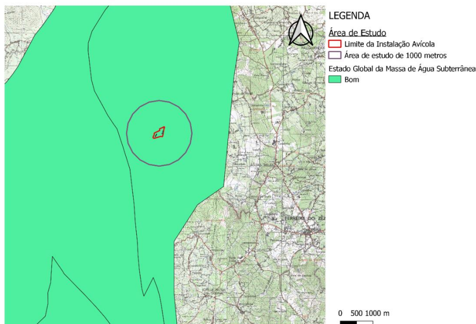
Figura 7.17 - Avaliação do estado global das massas de água subterrâneas (Fonte: PGRH RH5A, 2016; SNIAmb)
