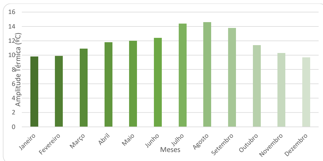
Figura 7.2 - Amplitude térmica registada na estação climatológica de Tancos/ Base Aérea (1951-1980)
