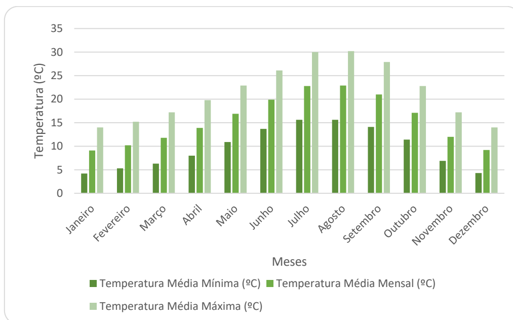
Figura 7.1 - Temperaturas mínimas, médias e máximas do ar, registados na estação climatológica de Tancos/ Base Aérea (1951-1980)
