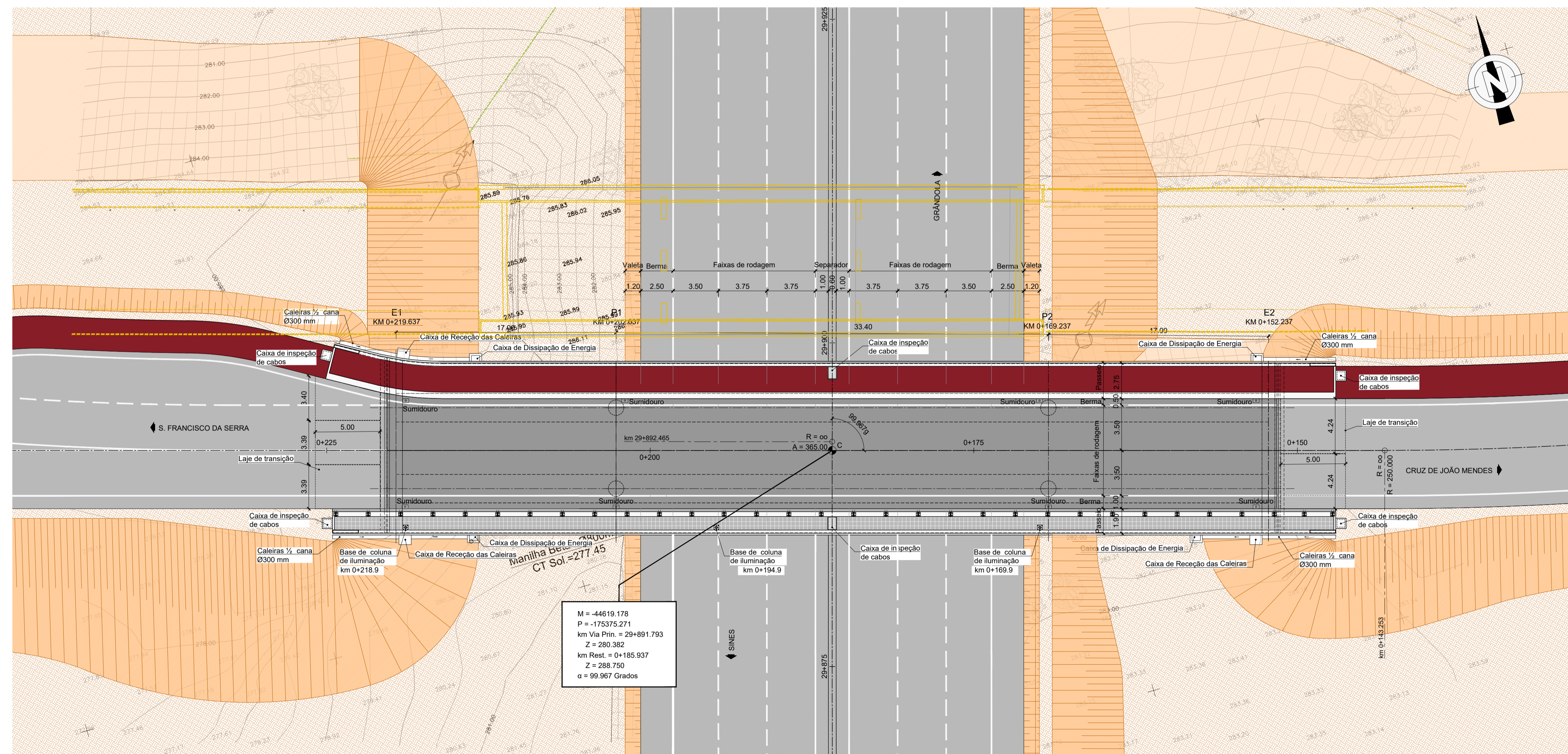
PLANTA ESC=1:200
